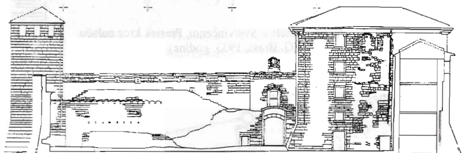
Fotogrametrijski snimak, 1983. - uzdužni presjek kroz kaštel.
