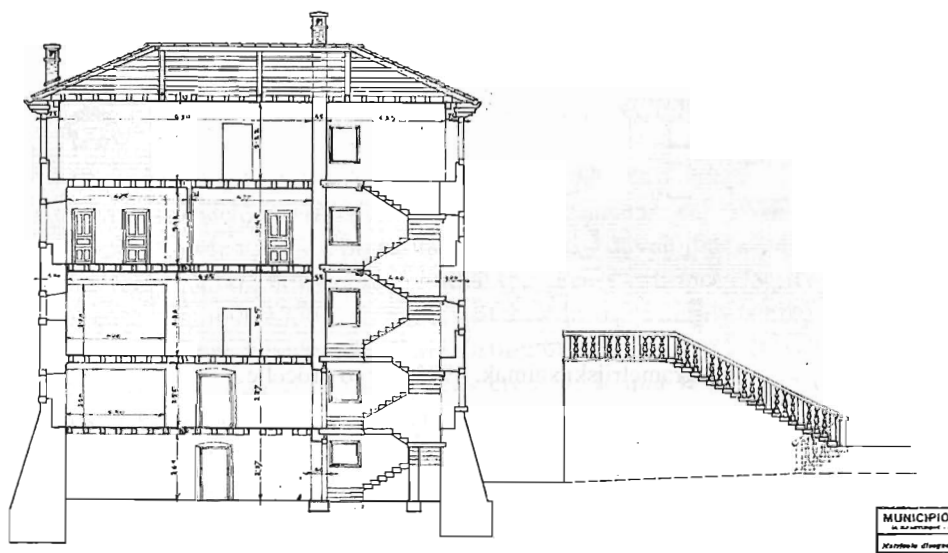
Projekt obnove kaštela u Svetvinčentu. Presjek kroz palaču. (G. Brass, 1933. godine)
