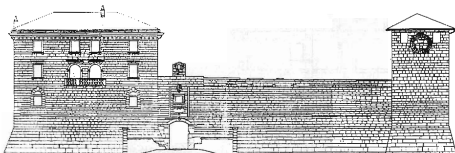
Fotogrametrijski snimak, 1983. južno pročelje.
