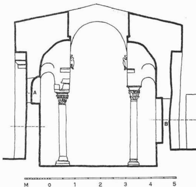
Sl. 5. Poprečni presjek kroz srednji travaj s pogledom na sjeverozapad (stanje 1957): A) Zazidan prozor, B) Zazidan portal. — Coupe transversale au milieu de la travée et vue sur le Nord-Ouest (état en 1957): A) Fenêtre murée, B) Portail muré
