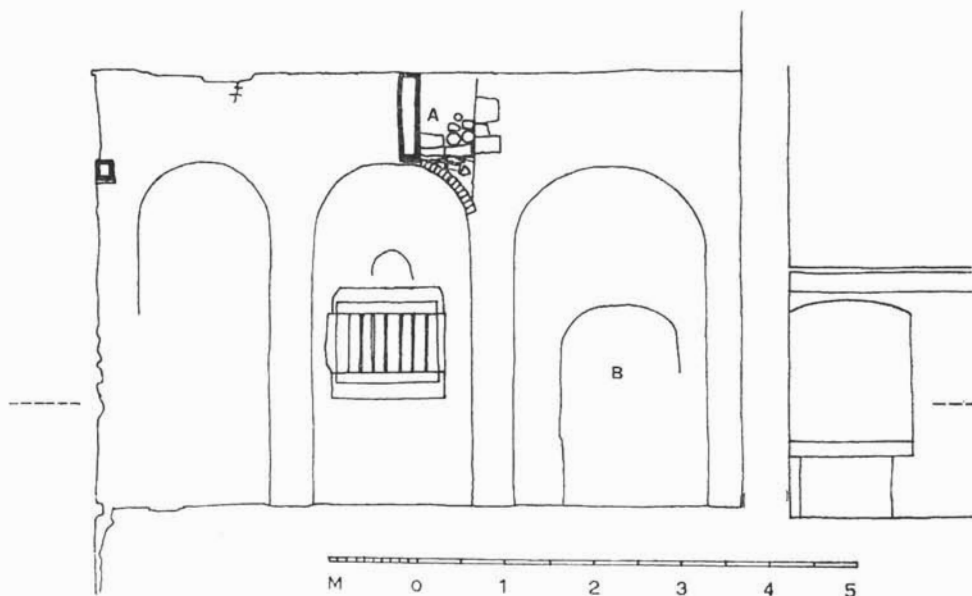
Sl. 13. Sjeveroistočni bočni zid (stanje 1957): A) Uzidani spoliji, B) Zazidan portal. — Mur latéral Nord-Est (état en 1957): A) Matériaux de rempli encastrés, B) Portail muré
