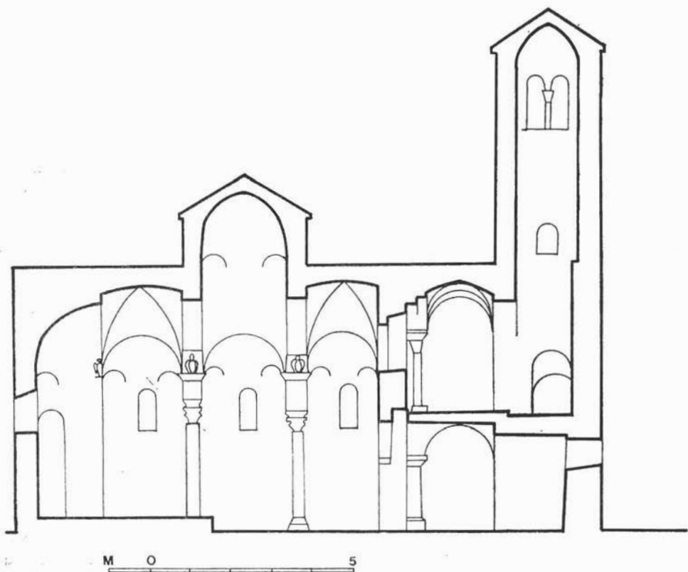
Sl. 15. Rekonstrukcija uzdužnog presjeka (pogled na jugozapad). — Reconstitution de la coupe longitudinale (vue vers le Sud-Ouest)
