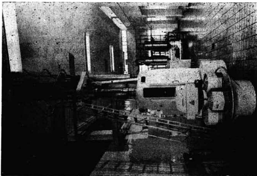
Linija za proizvodnju uperiziranog mlijeka u mljekari Sarajevo
