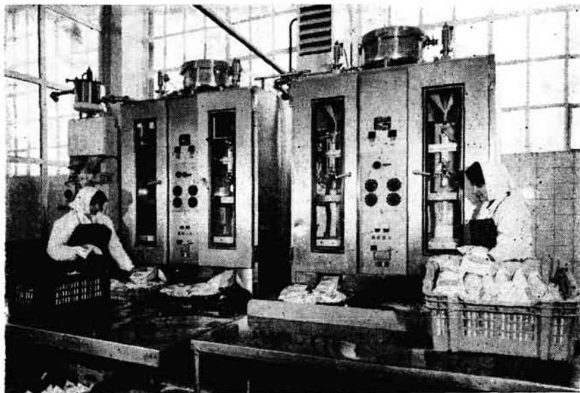
Strojevi PREPAC IS 5 za punjenje pasteuriziranog mlijeka kapaciteta 5000 l/h u mljekari Sarajevo
