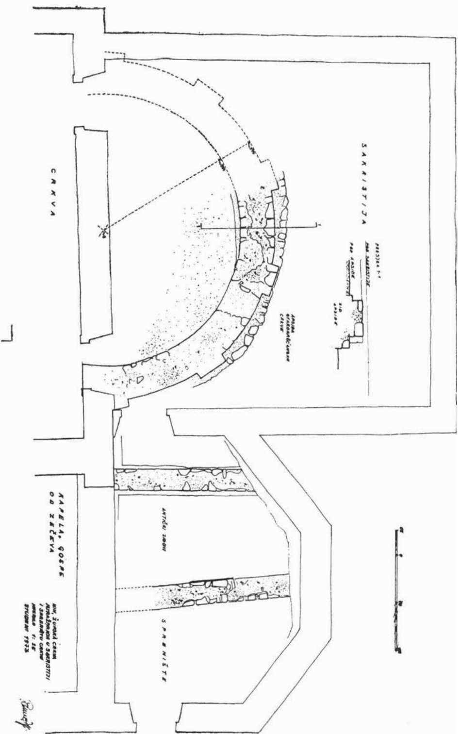
Crtež 3. Sakristija župne crkve u Nišu, tlocrt s ucrtanim ostacima starokršćanske apside. — La sacristie de l'église paroissiale de Niš, plan où sont indiqués les vestiges de l'abside paléochrétienne
