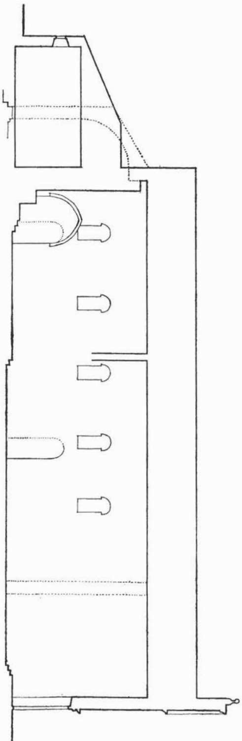
Crtež 7. Župna crkva u Ninu, uzdužni presjek s pogledom na južni zid. — L'église paroissiale de Nin, coupe longitudinale et vue sur le mur Sud
