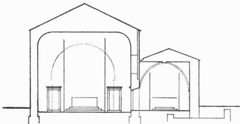
Crtež 9. Župna crkva u Ninu, poprečni presjek kroz crkvu i kapelu. — L'église paroissiale de Nin, coupe transversale à travers l'église et la chapelle
