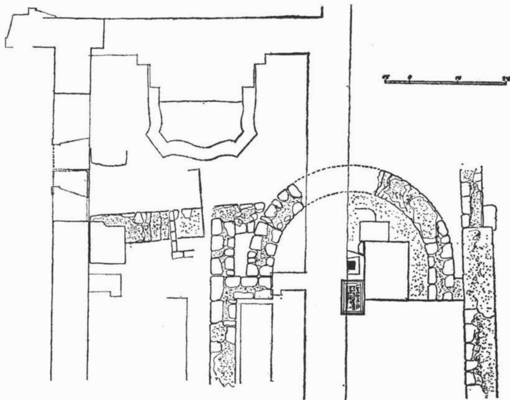
Crtež 4. Kapela župne crkve u Ninu, tlocrt s ucrtanim ostacima svetišta manje starokršćanske crkve. — La chapelle de l'église paroissiale de Nin, plan où sont indiqués les vestiges du sanctuaire de l'église paléo-chrétienne plus petite
