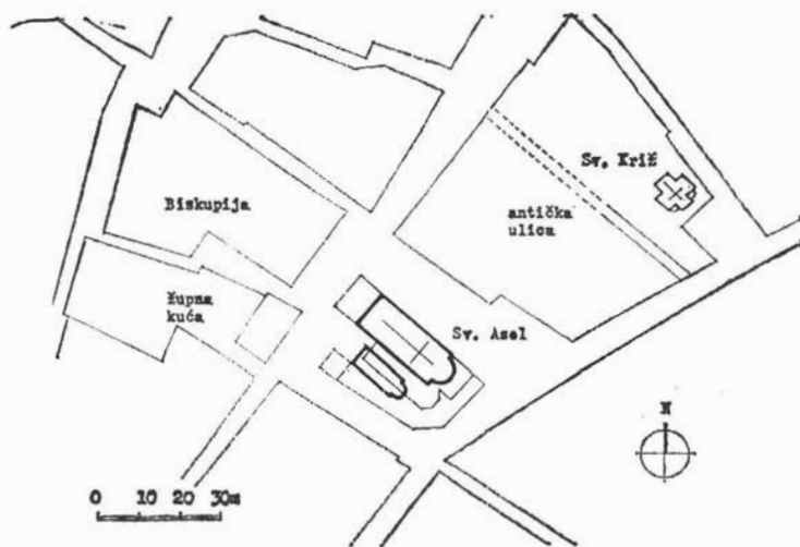
Crtež 1. Nin, sklop župne crkve, položajni nacrt. — Nin, ensemble de l'église paroissiale, plan de sa position
