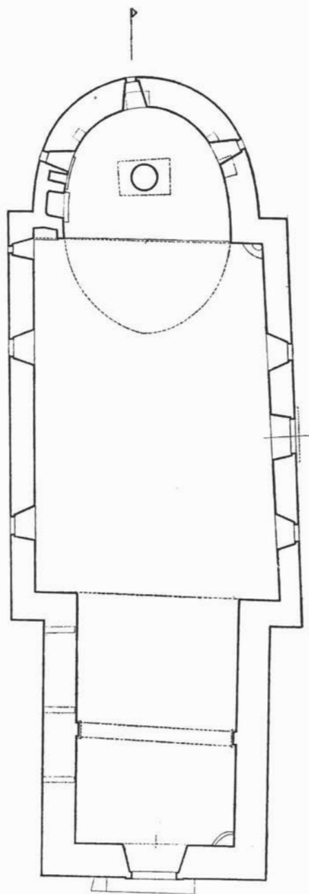
Biljane Gornje — Tlocrt crkvice sv. Jurja. M. 1:50. Arh. snimak: Medvedec — — Stepinac
