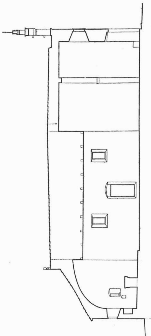
Biljane Gornje — Poprečni presjek crkvice sv. Jurja. M. 1:50. — Arh. snimak: Medvedec — Stepinac
