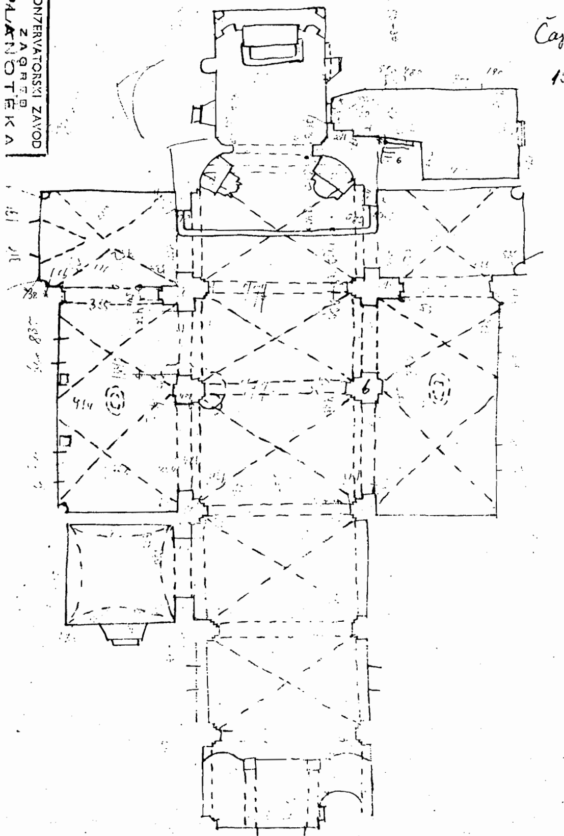
Tlocrt župne (nekoć dominikanske) crkve sv. Magdalene u Čazmi. Sagrađena je u XIII. stoljeću u gotičkom stilu, ali je nakon oslobođenja Čazme od Turaka barokizirana. (Planoteka Konzervatorskog zavoda u Zagrebu)
