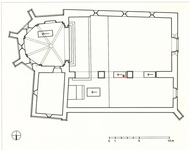
Slika 5. Požega, sv. Lovro. Tlocrt idealne rekonstrukcije gotičko-renesansne faze (Srša, 2005.).
