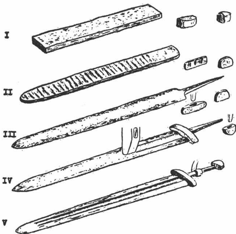
Sl. 1. Rekonstrukcija slijeda kovanja mača (tip X). — Abb. 1. Rekonstruierte Folge des Schwert-Schmiedeverfahrens (Typ X)
