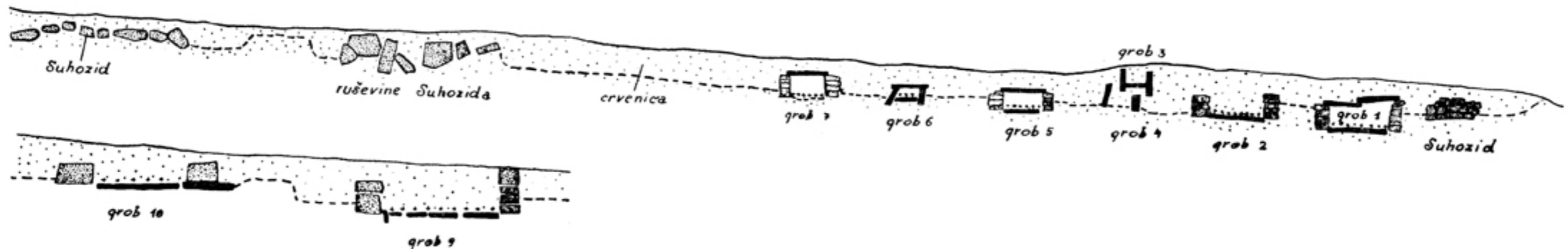
Crtež 3. Francini. Presjek c-d
