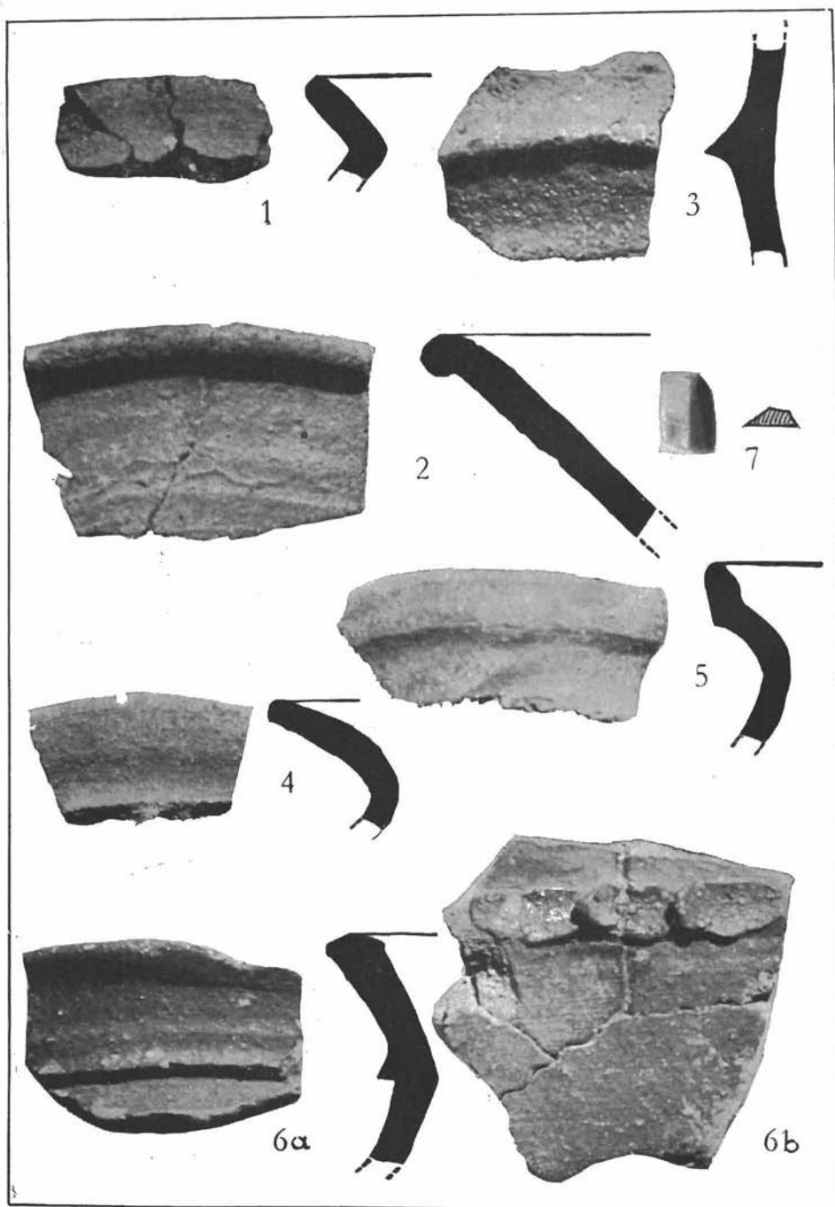
1 i 2. Sv. Mikula; 3-7. Sv. Lucija. Mjerilo 1 : 1.
