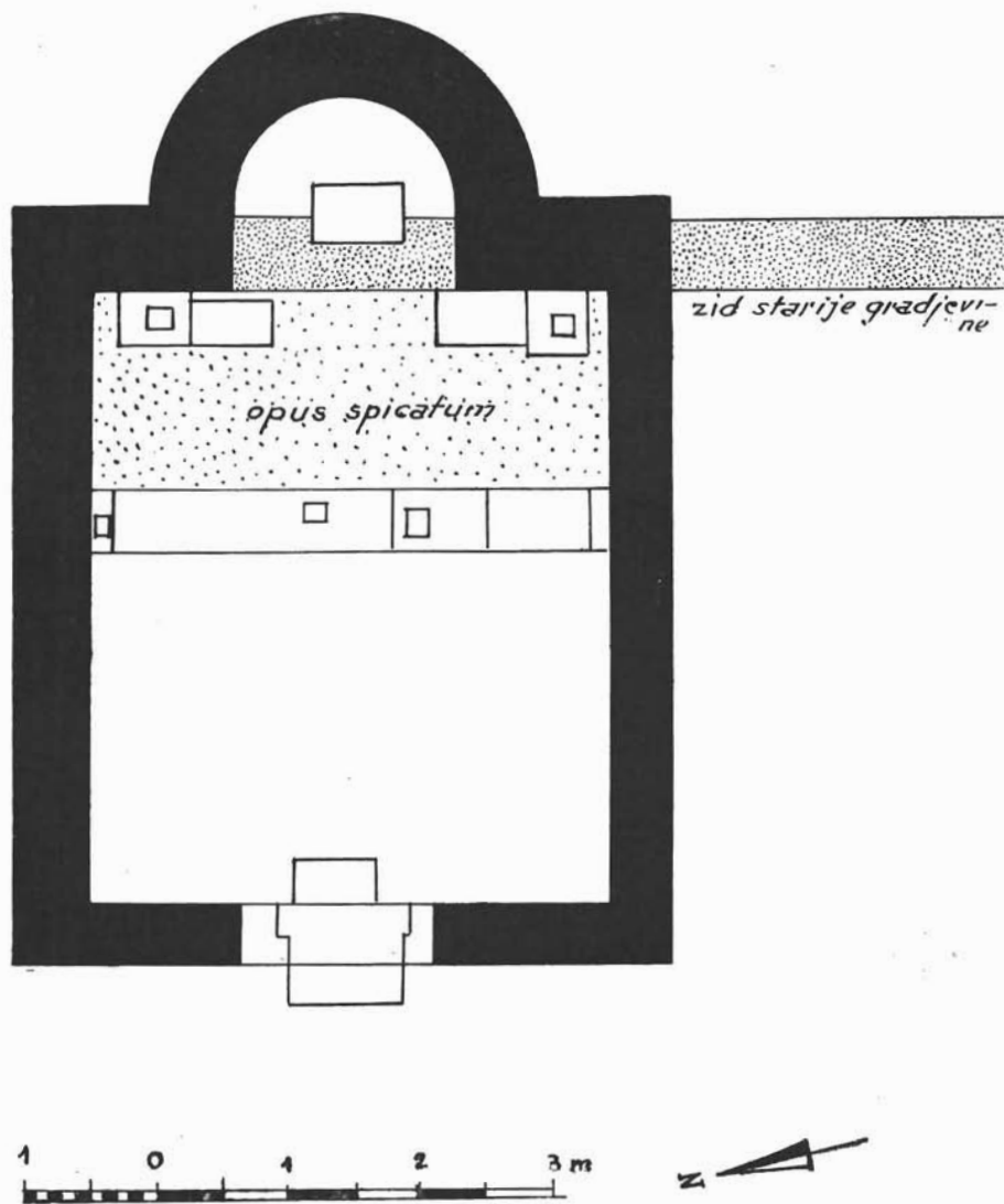
Sl. 3. Midnjan. Tlocrt romaničke crkve sv. Martina.
