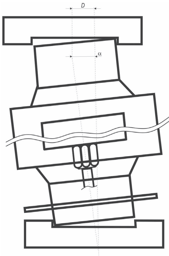
Slika 6. Prikaz najvećega otklona mjernoga pretvornika D = 18,5 mm, \alpha = 7^\circ
