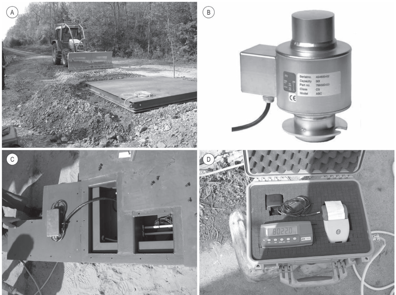
Slika 4. Prijenosna mjerna platforma i njezini sastavni dijelovi Fig 4. Portable measuring platform and its components
