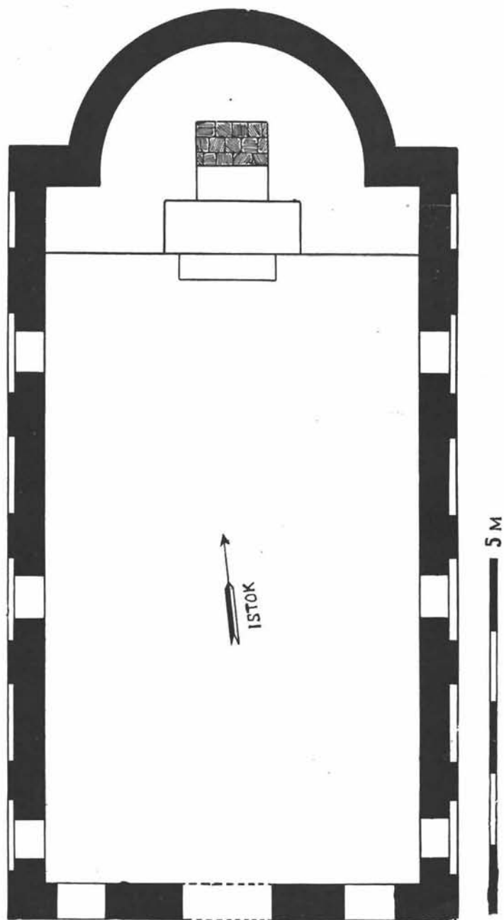
Sl. 15. Tlocrt crkve sv. Krištofa kod Rovinja
