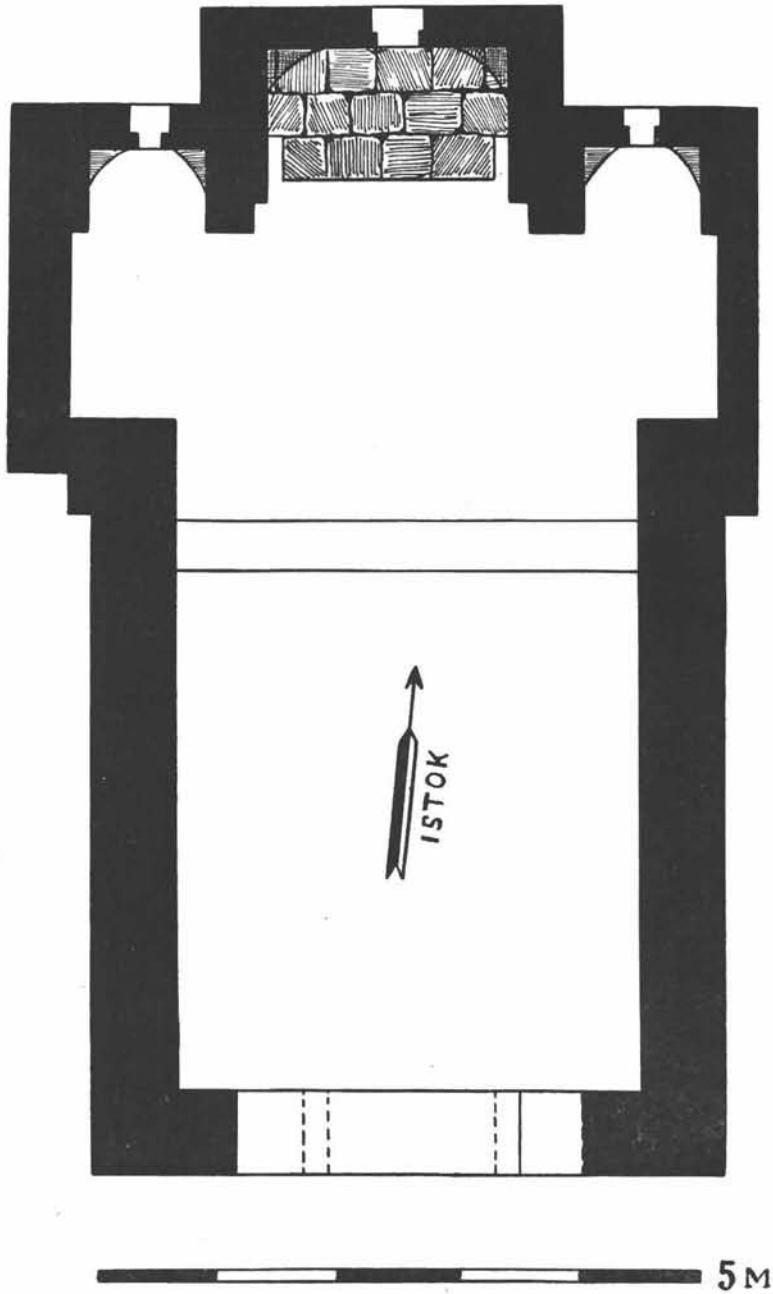
Sl. 18. Tlocrt crkve sv. Fume kod Rovinja
