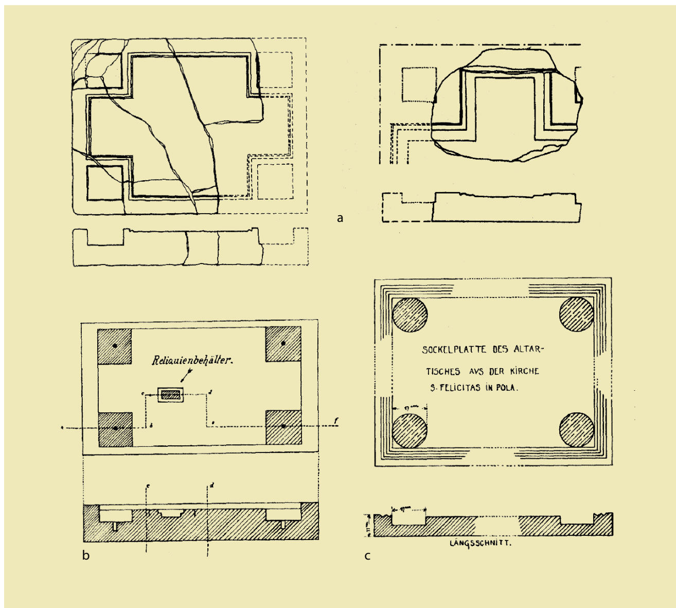
38. Primjeri baza oltara iz Istre: a) Eufrazijana u Poreču (izvor: CHEVALIER, P., 1999., 106), b) Sv. Marija na Brijunima, c) Sv. Felicitas (Sv. Ivan) u Puli [izvor: GNIRS, A. 2009., 212 (izvorno objavljeno: GNIRS, A., 1911.)]
