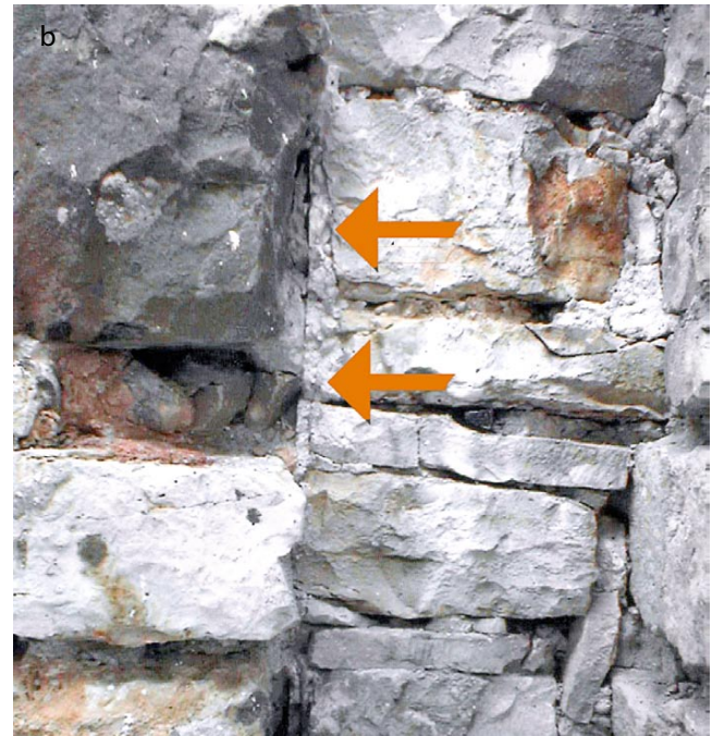
31. Istražno sondiranje, a) sonda na zidu u unutrašnjosti apside: 1. kamena građa zida, 2. prvi sloj žbuke, 3. nalič na prvom sloju, 4. drugi sloj žbuke, 5. dva ili tri sloja naliča; b) sonda na spoju zida priprate i jugozapadne lezene na pročelju crkve; c) unutrašnjost apside s konzerviranim i prezentiranim fragmentima izvorne pokrovne žbuke
