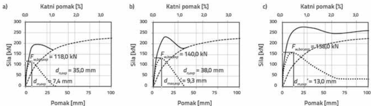
Slika 10. Doprinos ispune nosivosti: a) nearmirana ispuna; b) slabo armirana ispuna (šipke u sljubicama); c) slabo armirana ispuna (mrežica u sloju žbuke)
