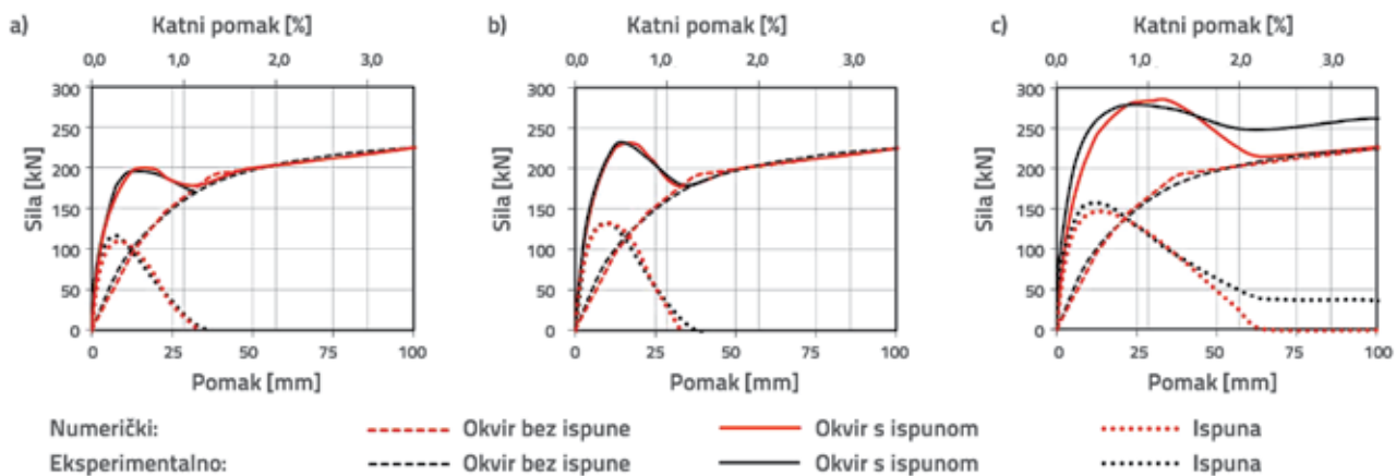
Slika 11. Usporedba numeričkih i eksperimentalnih rezultata: a) nearmirana ispuna; b) slabo armirana ispuna (šipke u sljubicama); c) slabo armirana ispuna (mrežica u sloju žbuke)
