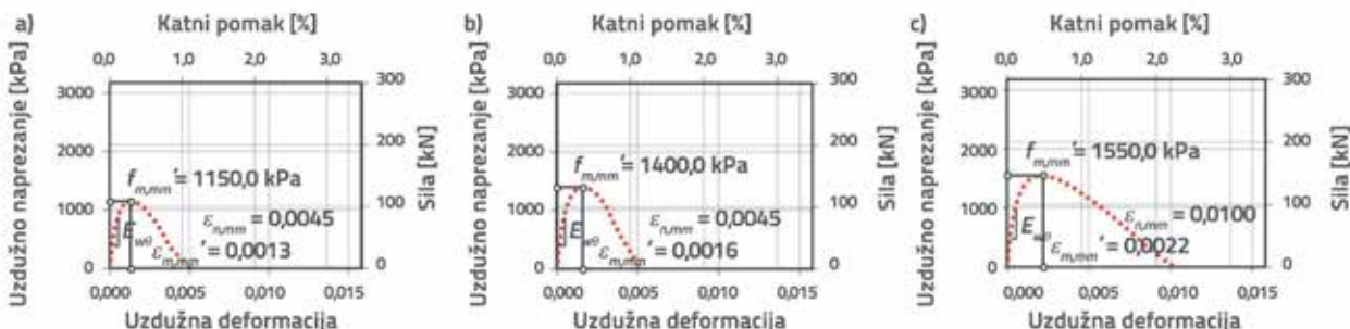
Slika 12. Dobivena ovisnost naprezanja i deformacija tlačne dijagonale: a) nearmirana ispuna; b) slabo armirana ispuna (šipke u sljubicama); c) slabo armirana ispuna (mrežica u sloju žbuke)
