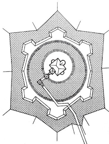
Slika 17. Konjščina, tlocrt kaštela i tvrđave (Zorislav Horvat i Krešimir Filipec, 2001.)
