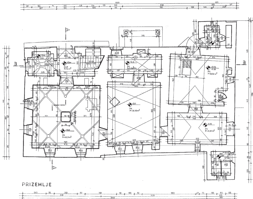
Slika 13. Ščrbinec, tlocrt prizemlja kurije (Ministarstvo kulture RH, Zagreb. Planoteka)
