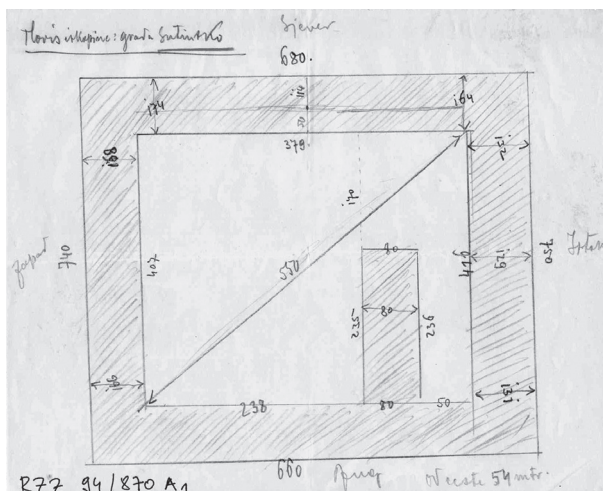
Slika 7. Sutinsko, skica tlocrta branič-kule kaštela iz 1910. (Ministarstvo kulture RH, Zagreb. Planoteka)
