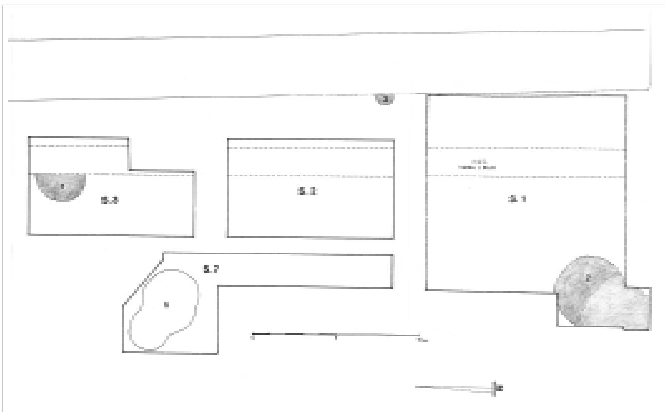
Sl. 1. Đakovo - Grabrovac, 1997. Horizontalni nacrt položaja ranobrončanodobnih jama (prema A. Durmanu)
