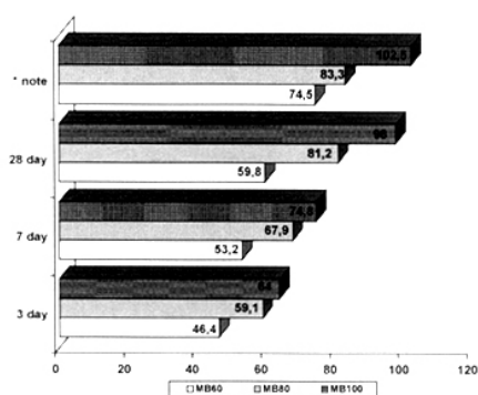
Slika 1. Ispitivanje tlačne čvrstoće betona (MPa) i rezultati dobiveni tijekom ispitivanja
