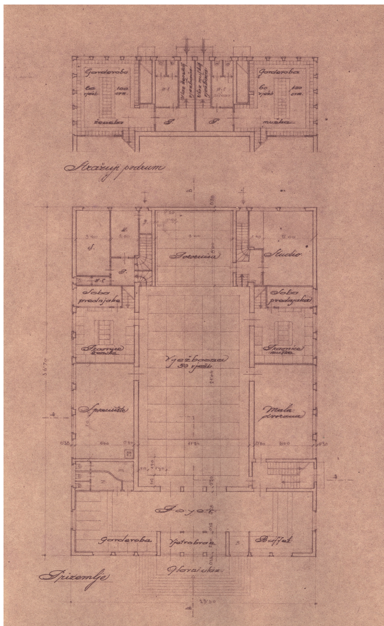
Slika 9. Projekt Sokolskog doma u Varaždinu (idejna skica) 26
