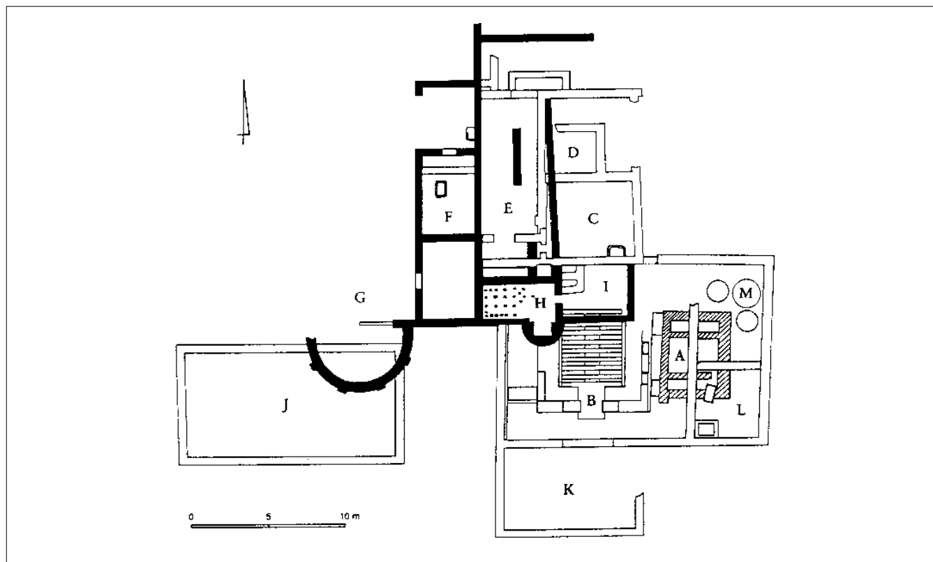
Sl. 9. Dvije istražene cjeline vile u Červar Portu kod Poreča (Girardi Jurkić, 1981.)
