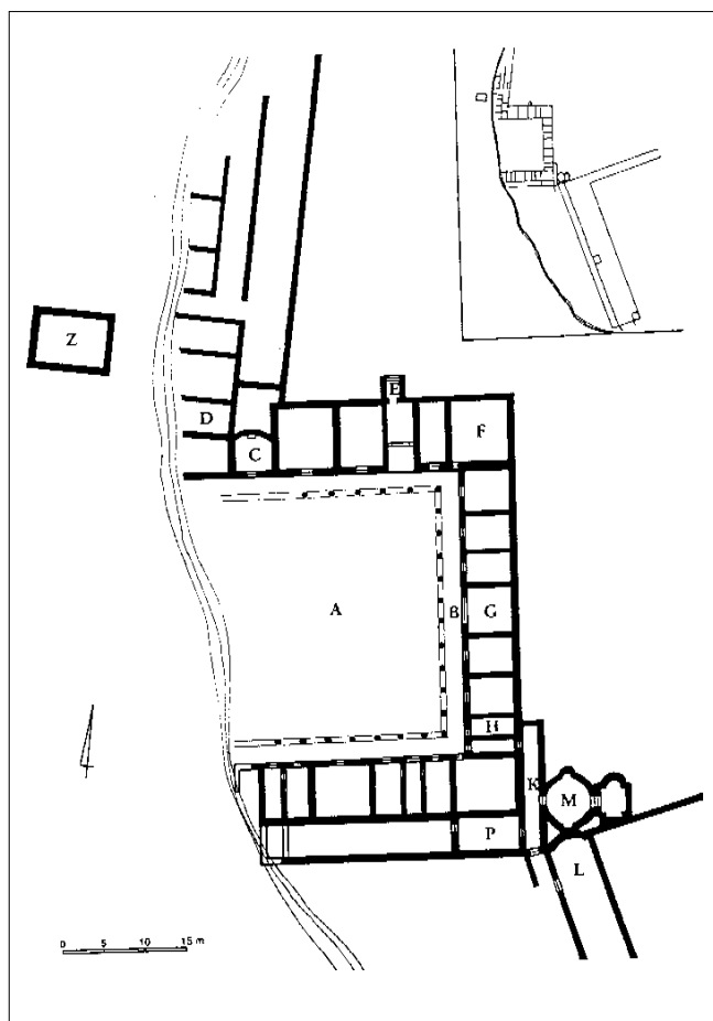
Sl. 2. Vila u Barbarigi (Schwalb, 1902.)
