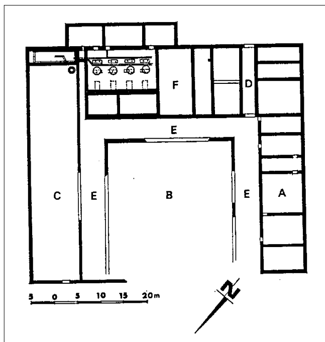
Sl. 4. Ostaci rustične vile na brdu Kolci, otočje Brijuni (Gnirs, 1908.)
