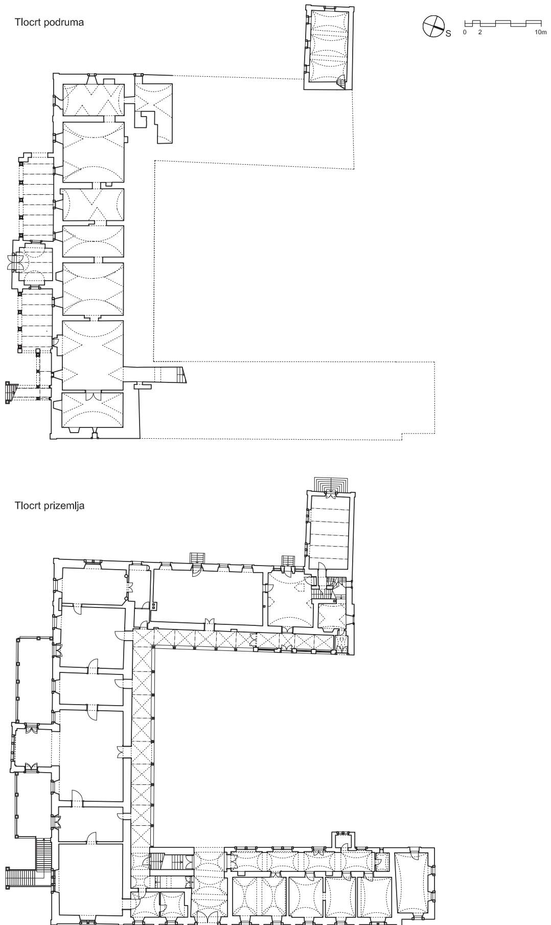
15. a,b. Tlocrt podruma, prizemlja, prvog i drugog kata te krovšta, prijedlog prezentacije (dokumentacija HRZ-a, izradili P. Puhmajer, M. Bogadi)
