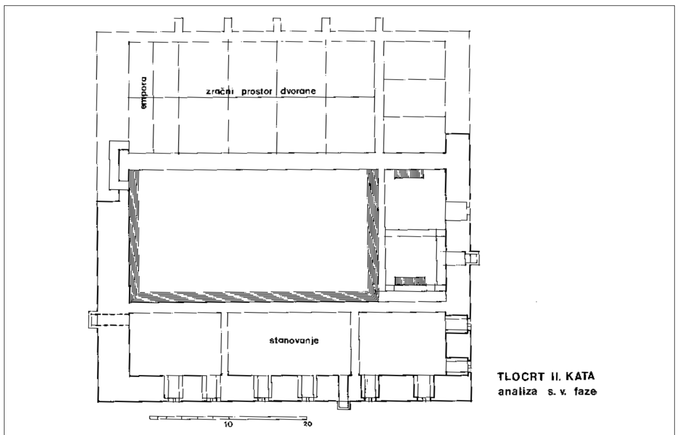
Abb. 12 Analyse des Grundrisses des Iločki-Palais, II. Stockwerk (gezeichnet von Z. Horvat nach der Vorlage des Fotos von B. Vučić und N. Škarić)
