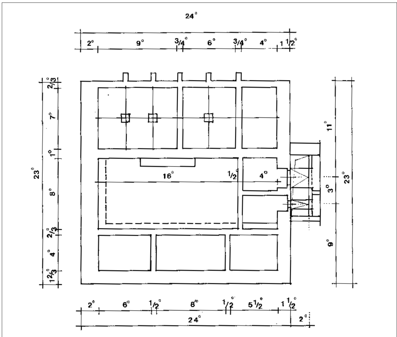
Sl. 13. Shema tlocrta palasa Iločkih, izražena u hvatima (1 hvat = 1° = 195 cm)
