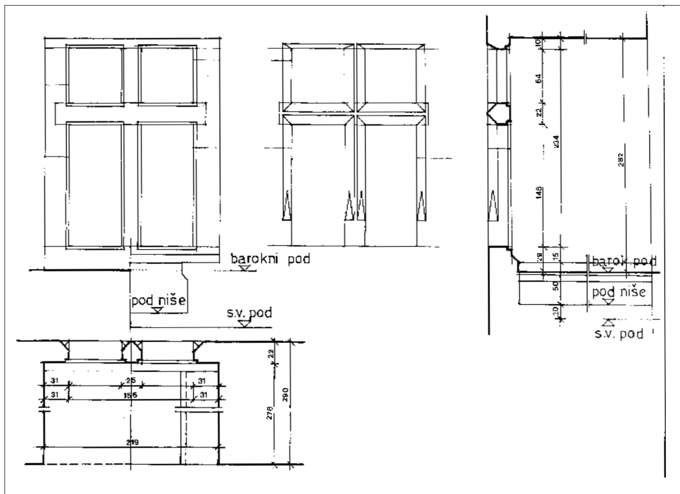
Sl. 16. Rekonstrukcija “češkog prozora” na II. katu palače Odescalchi - sl. 15.
