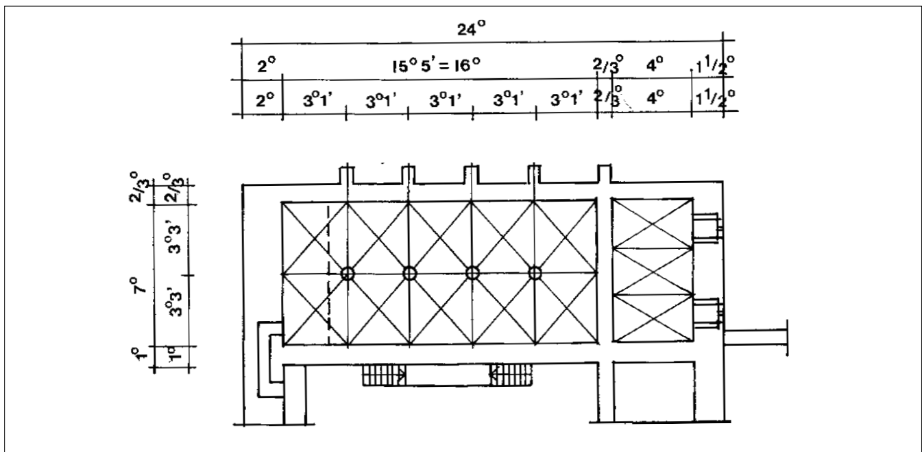
Sl. 14. Shema tlocrta viteške dvorane u sjevernom krilu palasa Iločkih, izražena u hvatima (1°) i stopama (1') (Z. Horvat)
