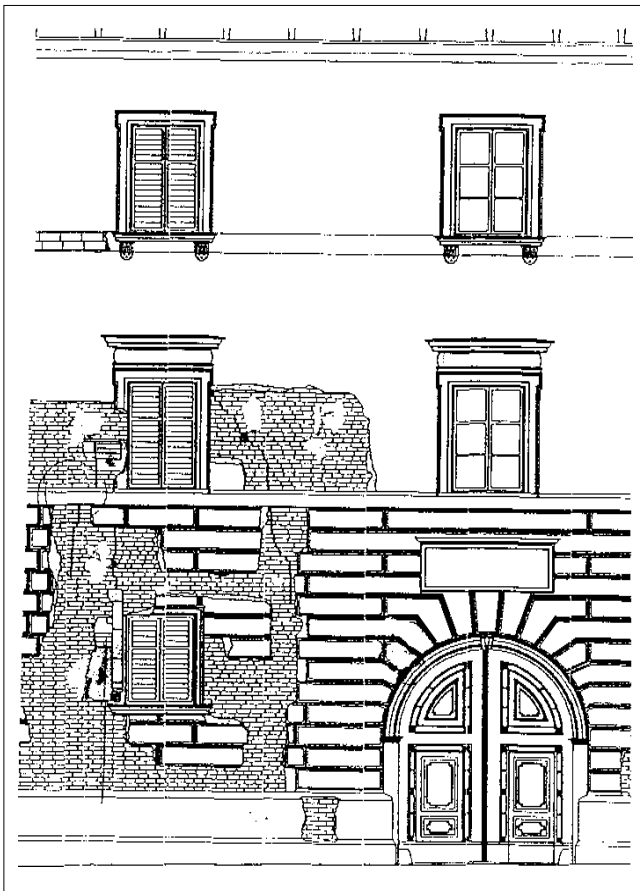
Sl. 19. Palača Odescalchi, istočno pročelje, detalj s nalazima ulaza za pješake palasa Iločkih (crtež B. Vučić i N. Škarić)
