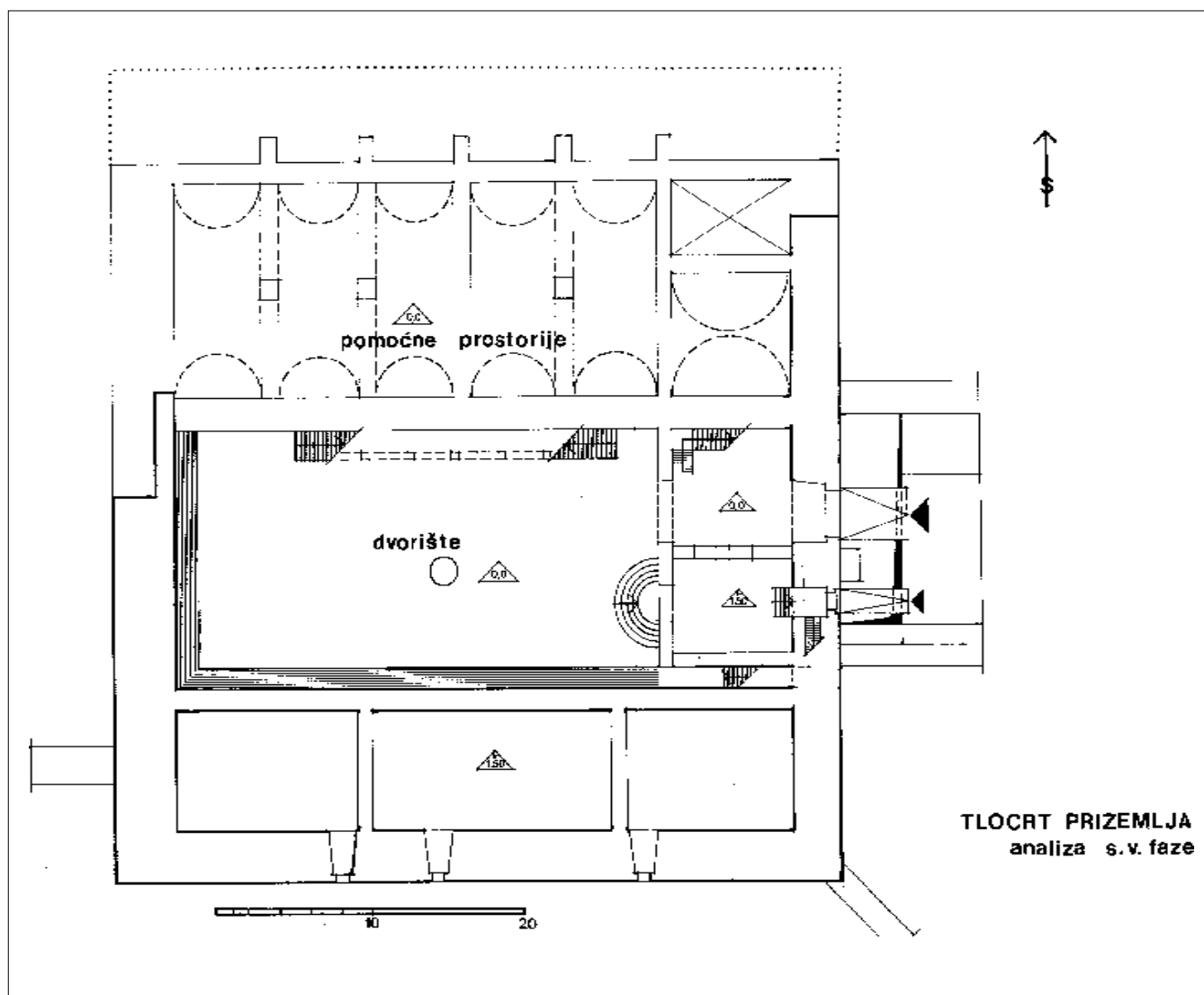
Sl. 10. Analiza tlocrta palasa Iločkih, tlocrt prizemlja (nacrtao Z. Horvat na podlozi snimaka B. Vučića i N. Škarića)
