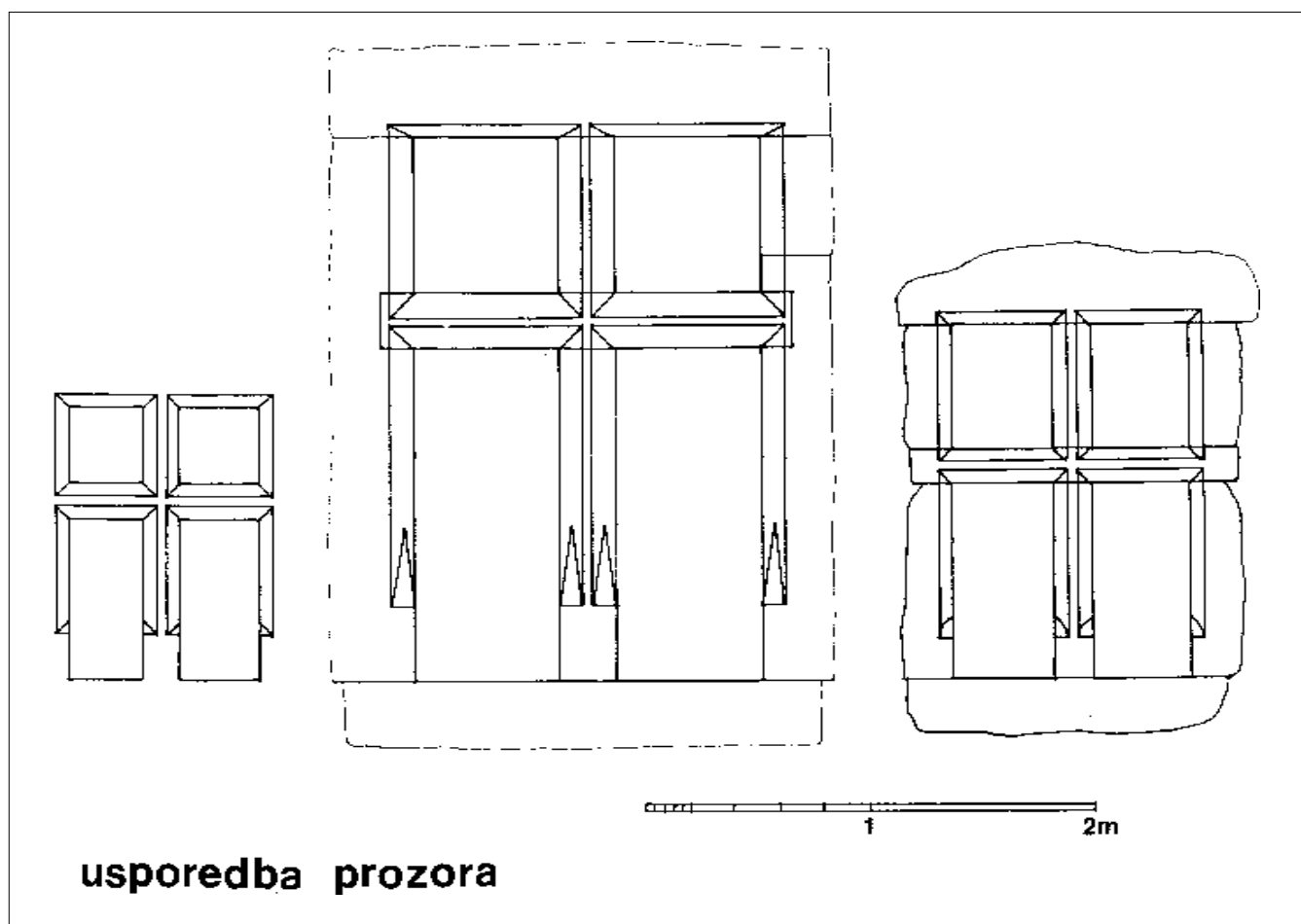
Sl. 18. Usporedni prikaz “čeških prozora” (lijevo - rekonstrukcija prozora sa srednje južne kvadratne kule u zidinama Iloka, sredina - II. kat palasa Iločkih, desno - “Žitnica”, Ozalj) (crtež Z. Horvat)
