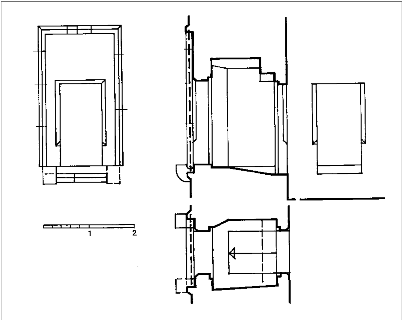
Sl. 21. Valpovo, ulaz na I. kat branič-kule (crtež Z. Horvat)
