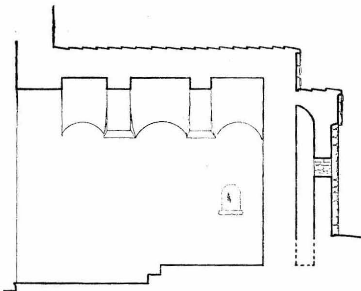
Sv. Ivan, Šipan: Uzdužni presjek
