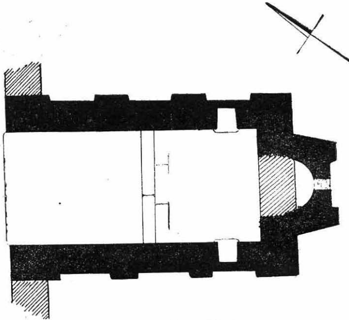
Sv. Ivan, Šipan: Tlocrt
