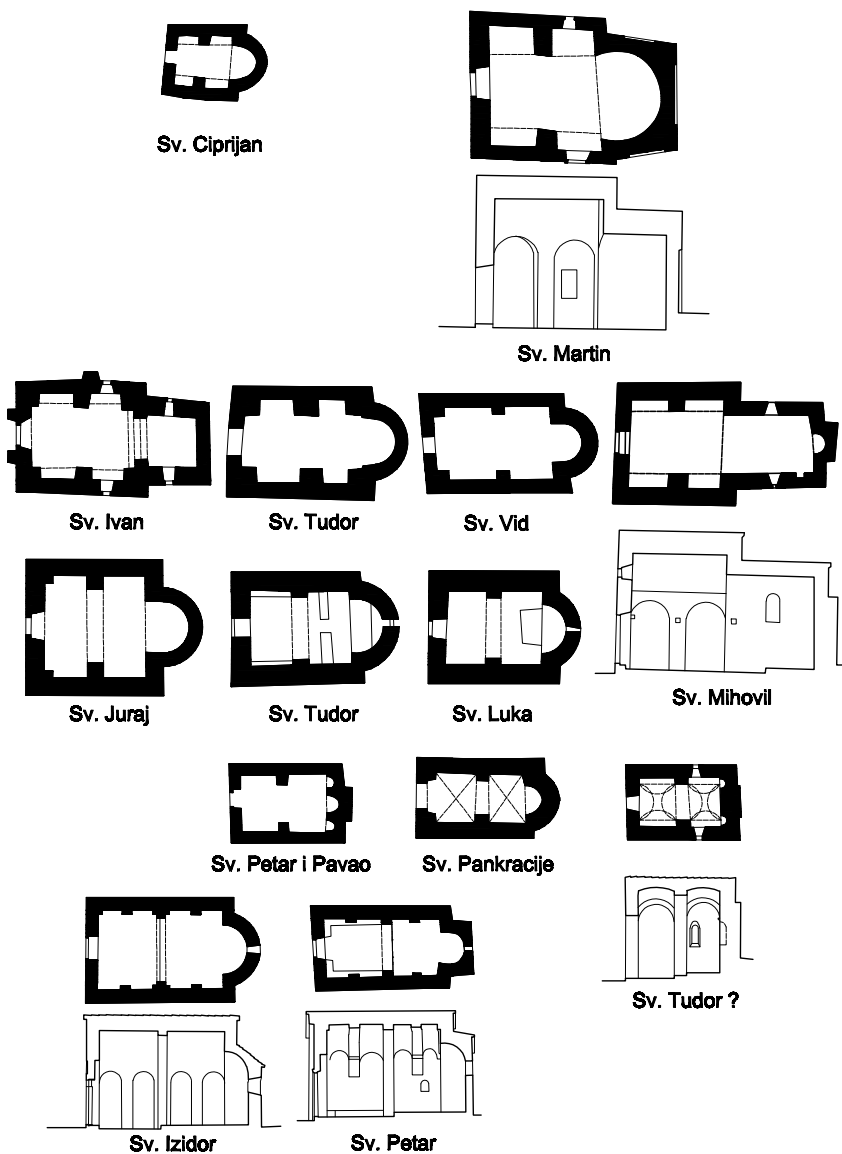
Tlocrti i presjeci ranosrednjovjekovnih crkava s dvodijelnom raščlanjenošću
