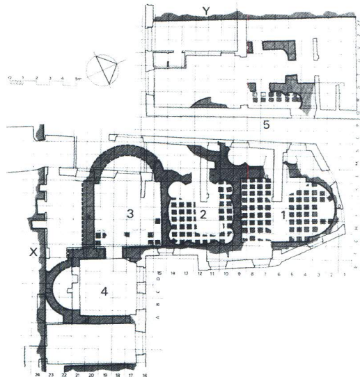
Tlocrt zapadnih termi neposredno izvan rezidencijalnog dijela Palače
