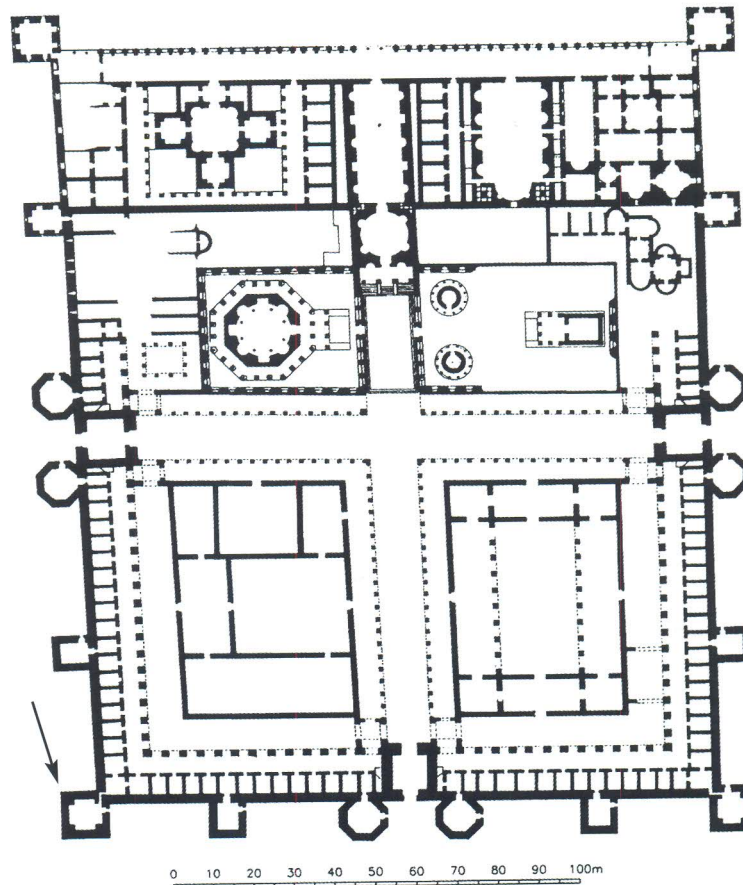
J. Marasović (1997), Tloclt Dioklecijanove palače, pretpostavljeno izvorno stanje
