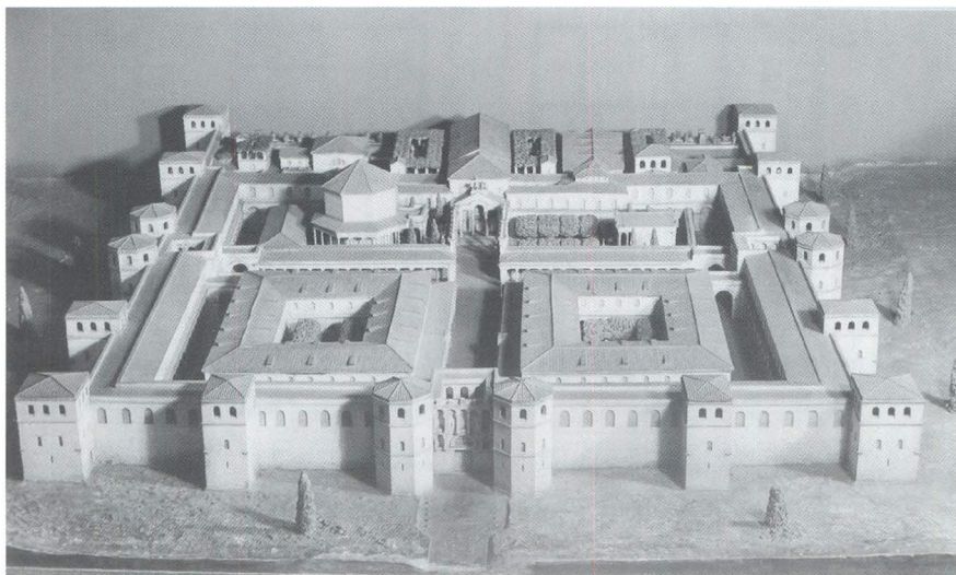
Model Dioklecijanove palače u pogledu preko dvaju blokova u sjevernom dijelu građevine, prema Hébrardovoj rekonstrukciji (1991)
