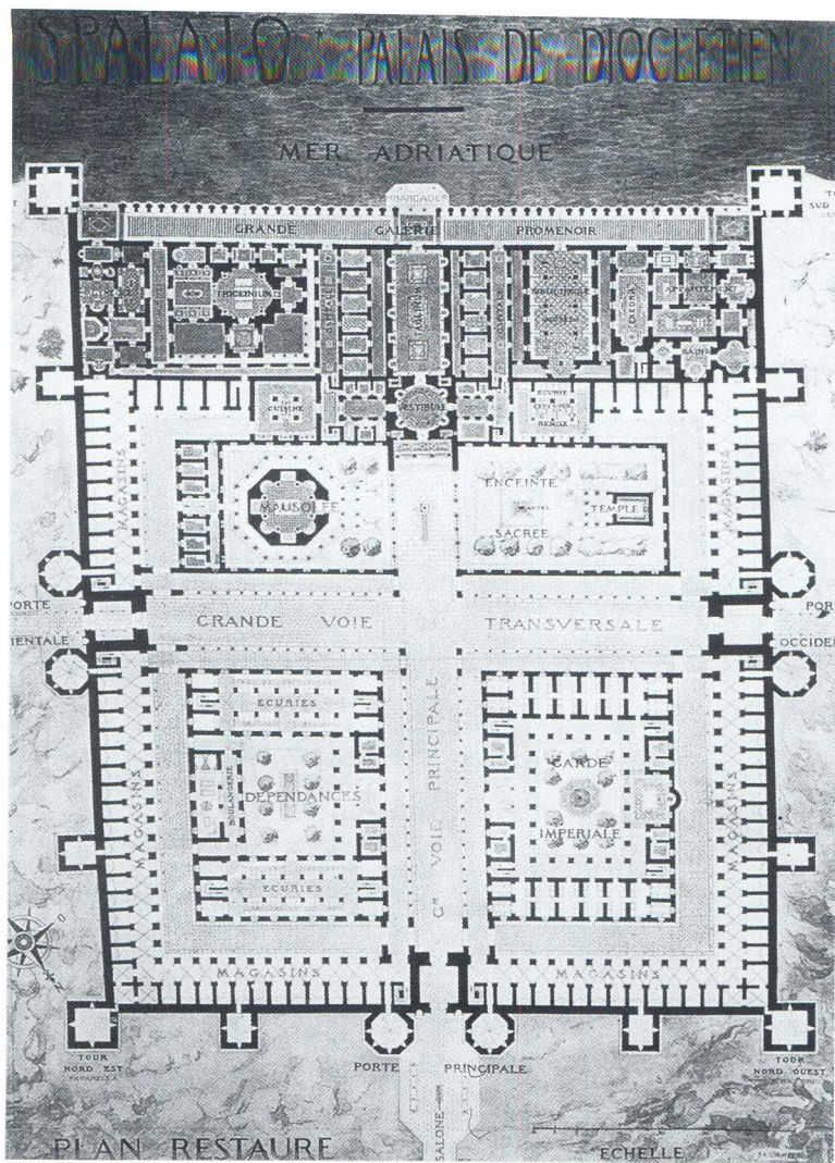
E. Hébrard, J. Zeiller (1912), Rekonstrukcija izvornog tlocrta Dioklecijanove palače (rezidencijalna zona naznačena je zatamnjeno; sjeverni blokovi su zamišljeni kao štale i prostori carske garde)
