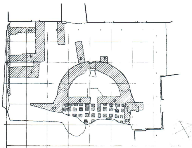
Tlocrt piscine i dijela hipokausta istočnih termi uz rezidencijalni dio Palače
