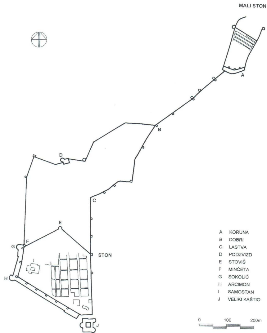
Stonski kompleks, shematski tlocrt (arh. I. Tenšek)
