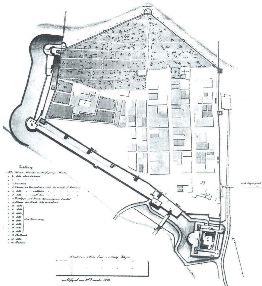
Ston, tlocrt, 1843. (Kriegsarchiv, Beč)
