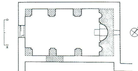
Tločrt crkve sv. Petra u Stonskom polju (prema I. Fiskoviću)
