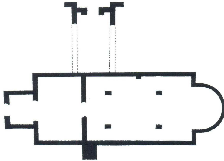
Tlocrt crkve u Žažviču (prema L. Marunu)
