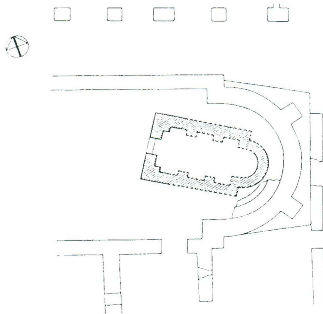
Tloert crkve sv. Petra u Ublima na Lastovu (prema I. Fiskoviću)
