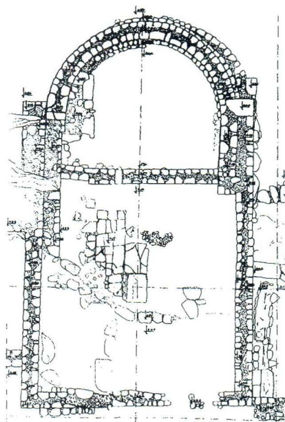
Tlocrt crkve u Rižinicama (Solin)
