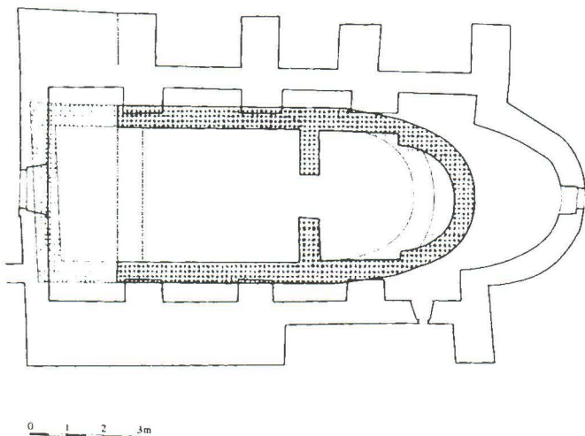
Tlocrt crkve sv. Silvestra na Biševu (prema I. Vojnoviću)
