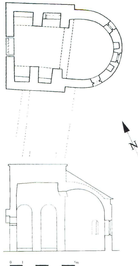
Tlocrt i presjek starokršćanske crkve sv. Stjepana u Pučišćima na Braču s reduciranim opsegom u ranom srednjem vijeku (prema R. Bužančiću)
