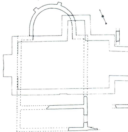
Tlocrt predromaničke crkve u Muću Gornjemu (prema M. Zekanu)
