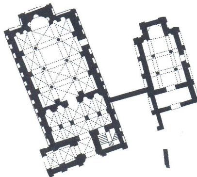
Razvoj srednjovjekovne crkve sv. Stjepana na Otoku: a) crkva 9. st., b) Jelenina obnova u drugoj polovici 10. st. i c) ranoromanička obnova u drugoj polovici 11. st.
