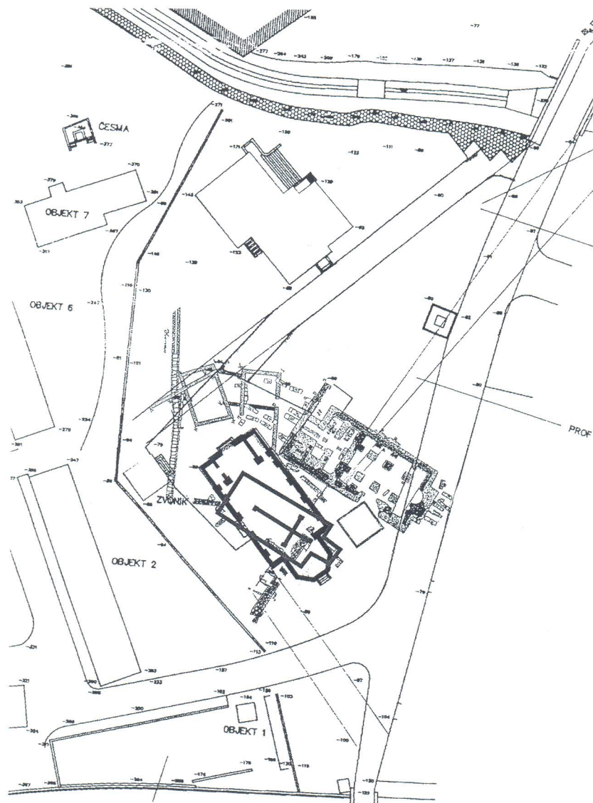
Položaj stare crkve Gospe od Otoka iz 1820. g. i arhitektonski snimci lokaliteta uneseni na geodetski snimak iz 1992. g.
