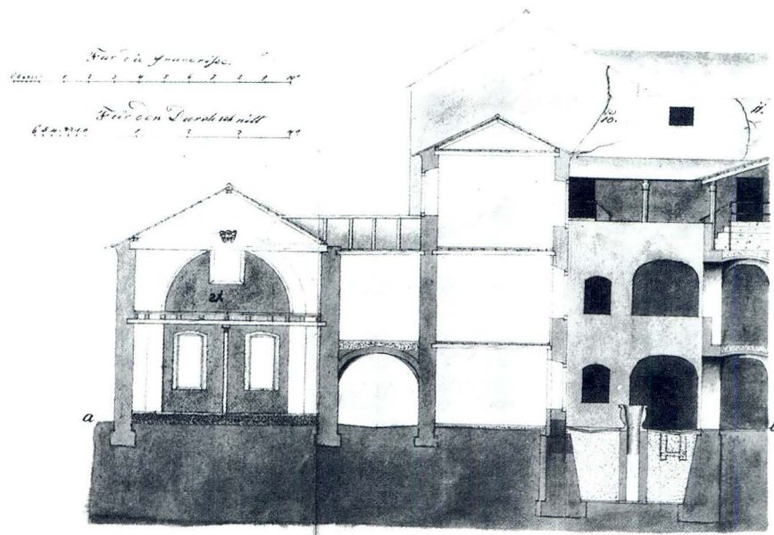
Poprečni presjek kroz crkvu i samostan sv. Marcele, izraden u vrijeme preuređenja u vojarnu 1828. godine. (Hrvatski državni arhiv - Zagreb)
