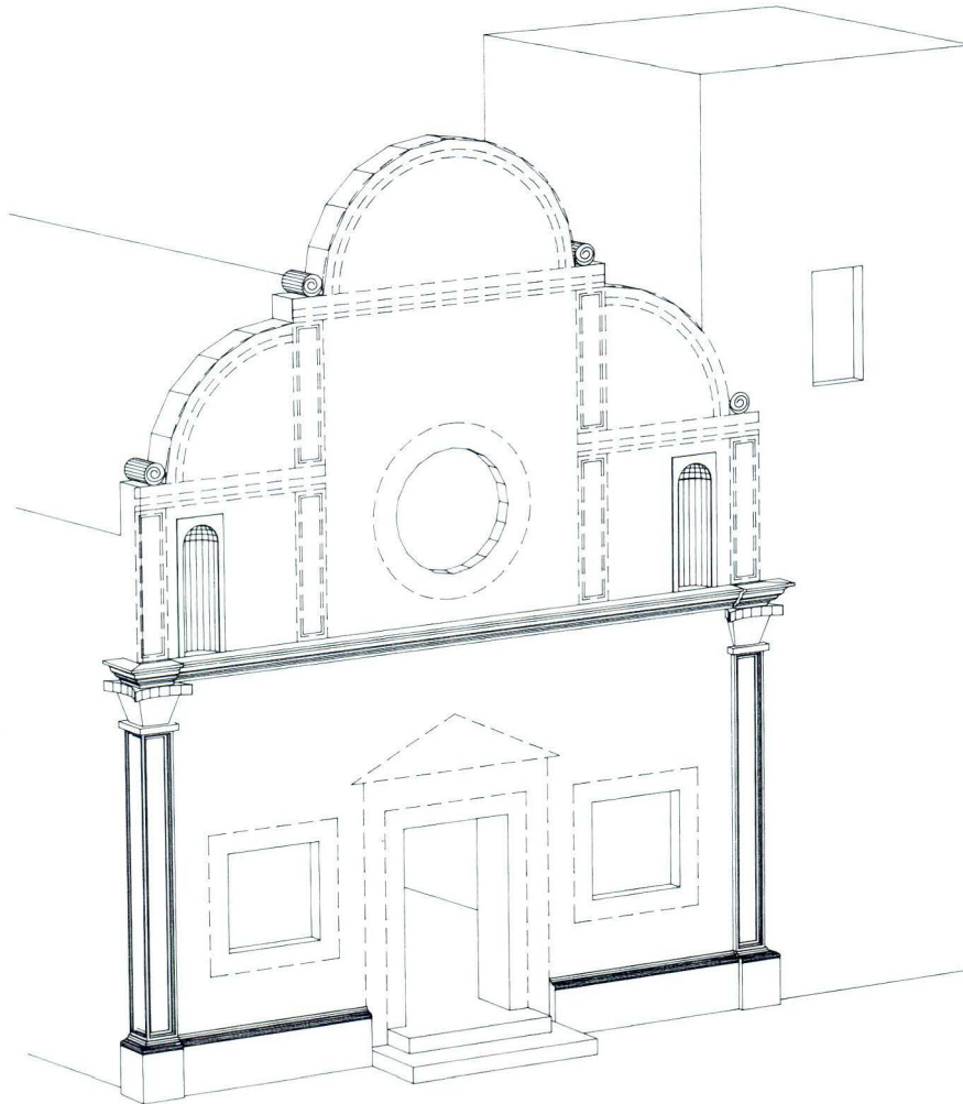
Pogled na pročelje i zvonik Sv. Marcele. Pune crte označavaju izvorno stanje napravljeno na temelju podataka iz arhivskih nacрта i sačuvane arhitektonske plastike. Crtkano je prikazan hipotetični izgled trilobnog pročelja i pretpostavljena profilacija prozora i vrata. (Kompjutorska izrada dipl. ing. arh. S. Štok)
