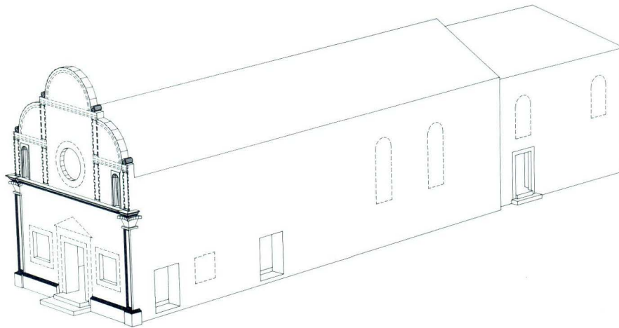
Kosa projekcija crkve sv. Marcele gledano s jugozapada. Dimenzije i oblici s nedostatnim podacima izrađeni su crtkano. (Kompjutorska izrada dipl. ing. arh. S. Štok)
