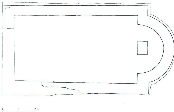
Tloris sv. Marine kod Zadra (P. Vežić)
