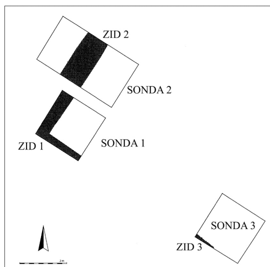
Sl. 15. Tlocrt otkrivenih zidova u sondama 1-3 (Arheolog d.o.o.)
