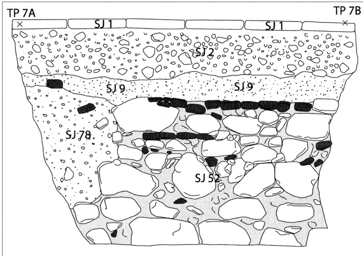
Sl. 16. Pogled na zid 3 unutar Sonde 3 (Arheolog d.o.o.)
