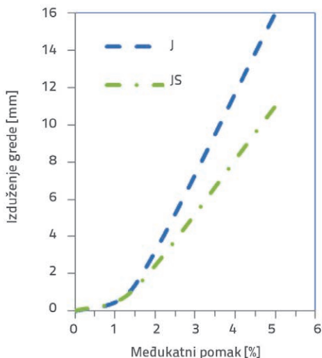
Slika 15. Izduženje/rasterećenje grede
