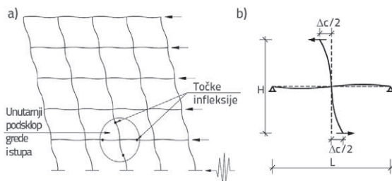
Slika 2. a) Prototip okvira pod utjecajem bočnog seizmičkog opterećenja; b) modeliranje unutarnjeg podsklopa grede i stupa
