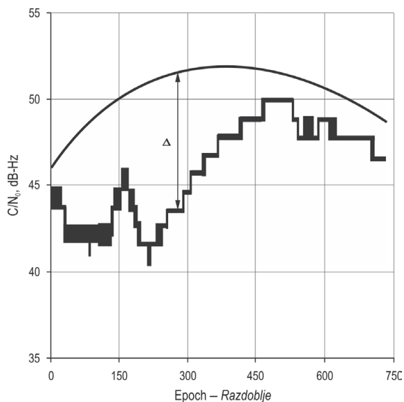
Fig. 9 C/N_0 values of L1 signal and template model ( \hat{\ }^ ) for the site T_2 Slika 9. C/N_0 vrijednosti signala L1 i predloženi model ( \hat{\ }^ ) za mjesto T_2
