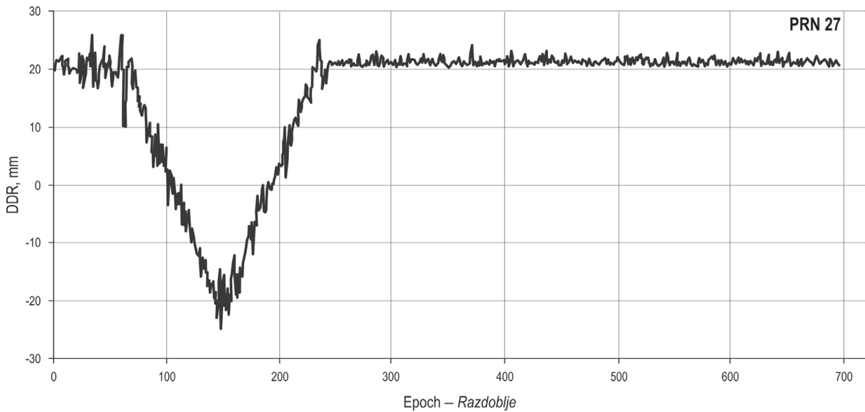
Fig. 7 Double difference residuals of PRN 27 for the baseline T_1-T_2 Slika 7. Dvostruki diferencijalni ostaci od PRN 27 za osnovnu liniju T_1-T_2
