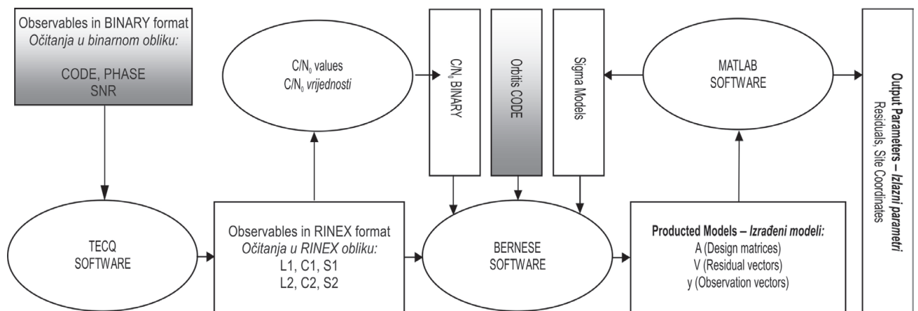
Fig. 4 Computing scheme: Inputs, algorithms, software programs and outputs Slika 4. Plan načina izračuna: ulazni podaci, algoritmi, računalni programi i izlazni podaci
