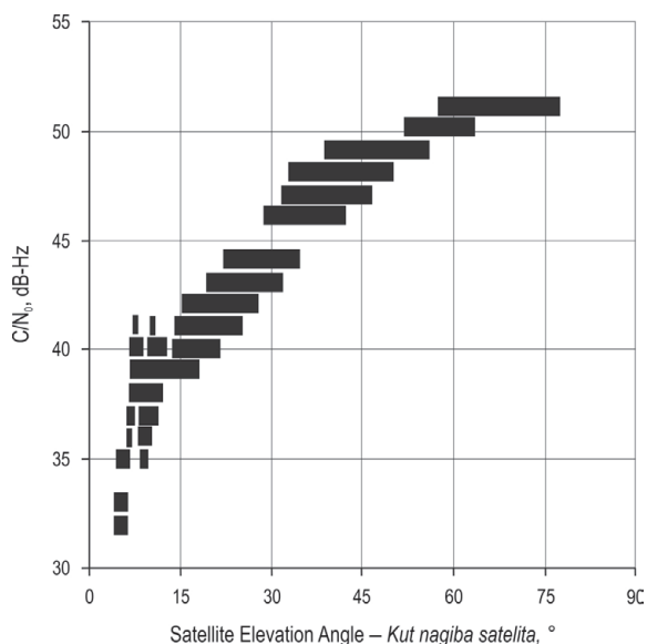
Fig. 8 C/N_0 values of L1 signal for the site T_1 Slika 8. C/N_0 vrijednosti signala L1 za mjesto T_1
