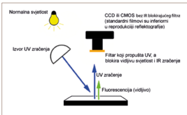
11 Shema snimanja UV reflektografije UV reflectography shooting scheme
