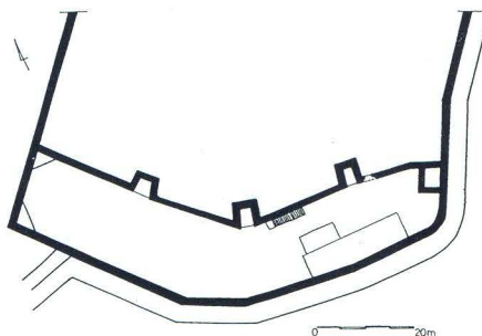
Tvrđava Koruna, Tlocrt 1450. godine
