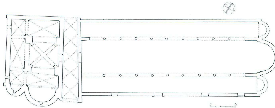
Krk, Katedrala sv. Marije i crkva sv. Kvirina, tlocrt /arh. snimak: I. Tenšek/
