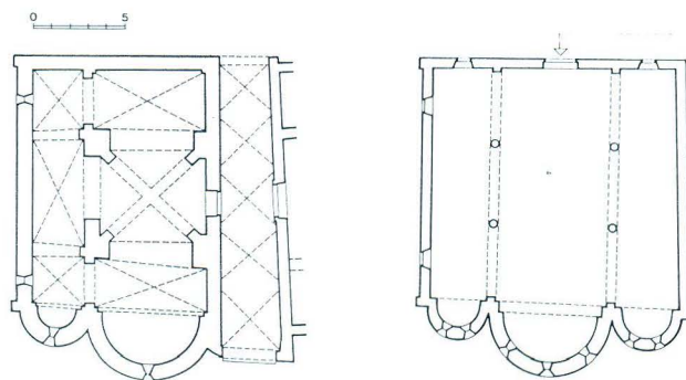
Krk, Sv. Kvirin, tlocrt prizemlja
