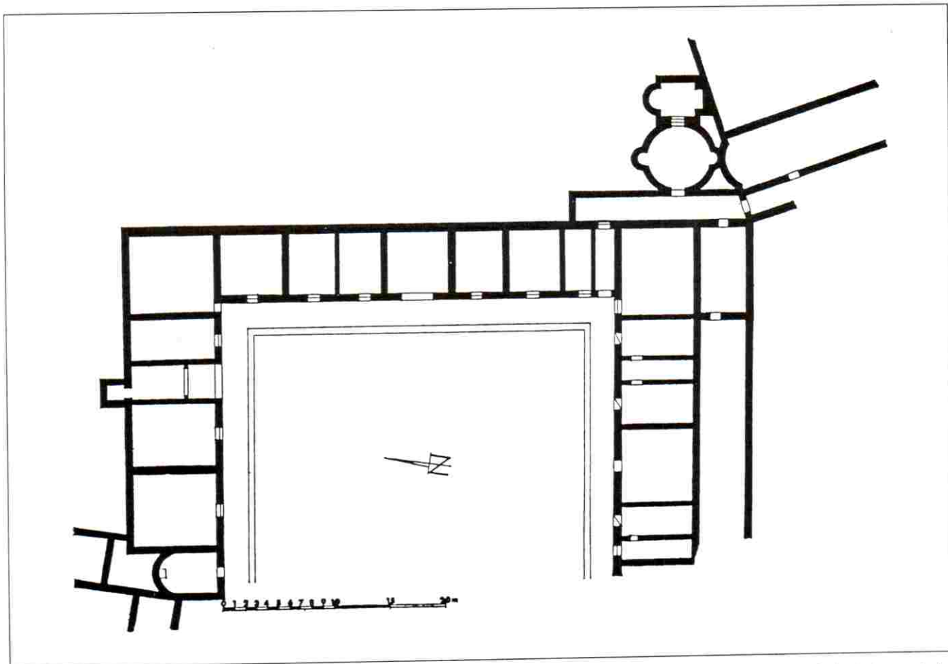
Sl. 1. Vila kod rta Barbarige u Istri (tlocrt prema GNIRS-u)
