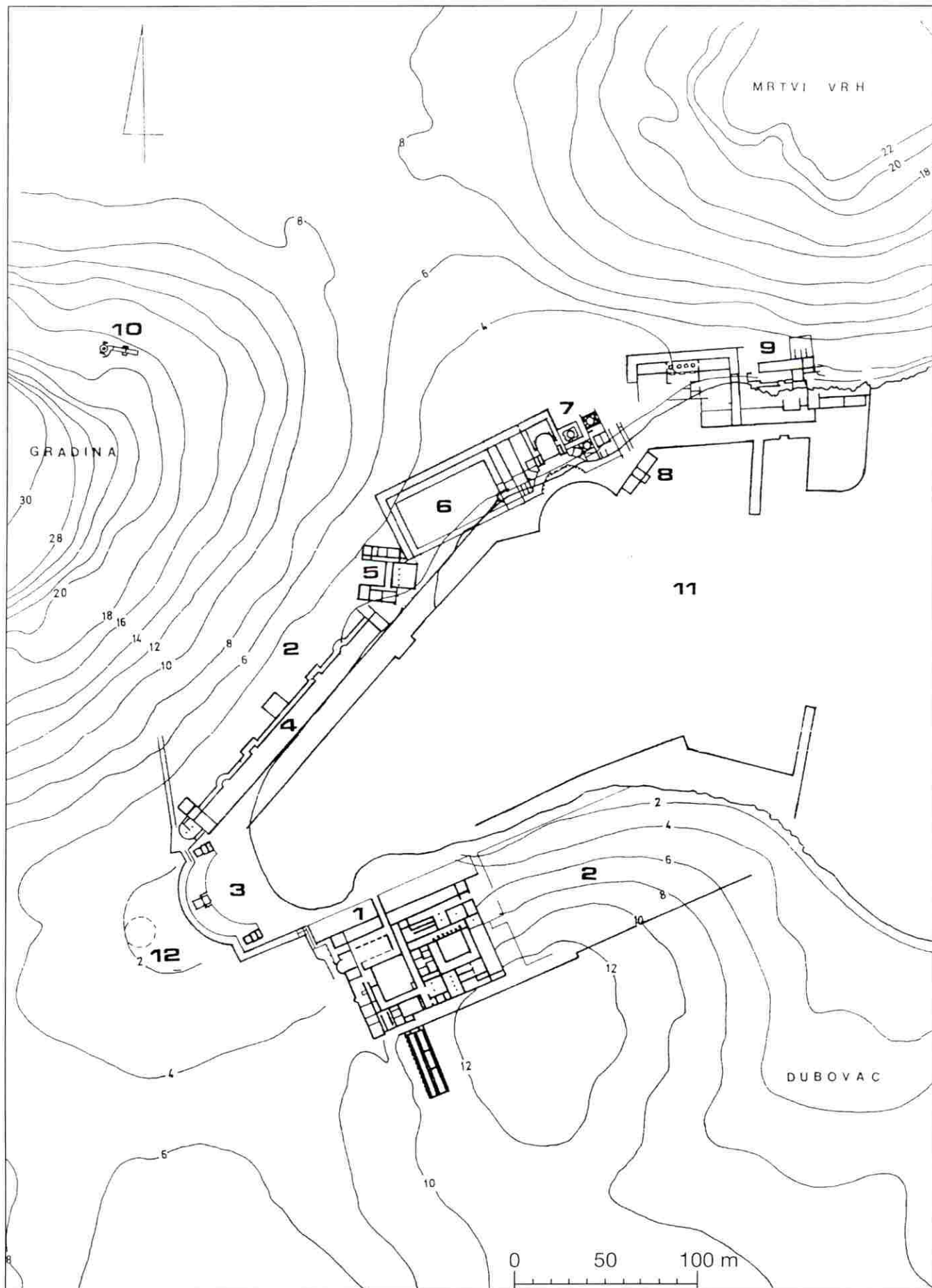
Sl. 6. Vila u rvali Verige na Brijunima (tlocrt prema BEGOVIĆ)
