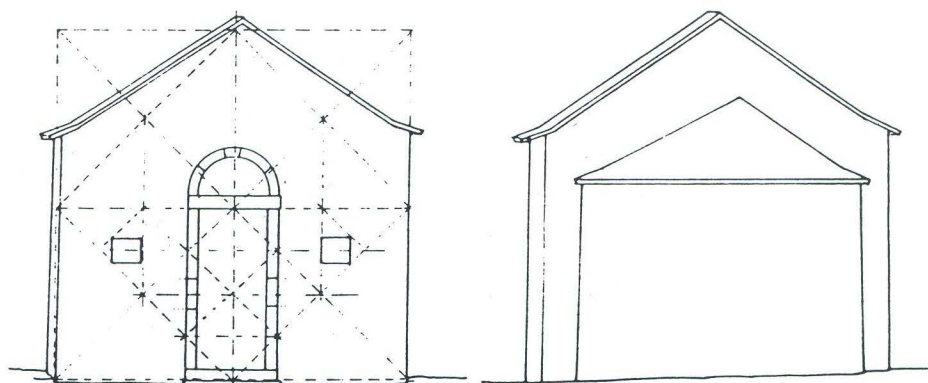
Tloct i presjeci crkve sv. Vida kod Grablja
