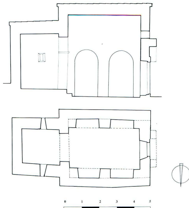
Izgled Sv. Ivana nakon ranosrednjovjekovnog preuređenja
