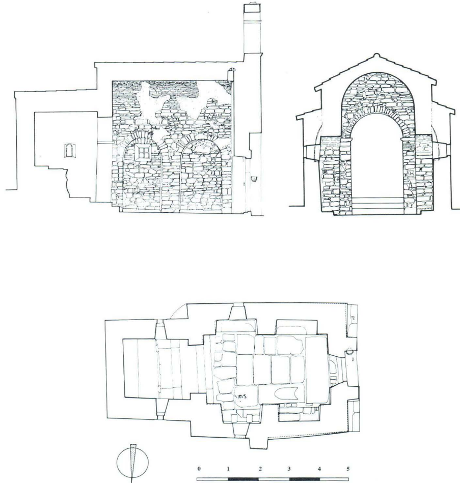
Sv. Ivan u Bolu, snimak postojećeg stanja
