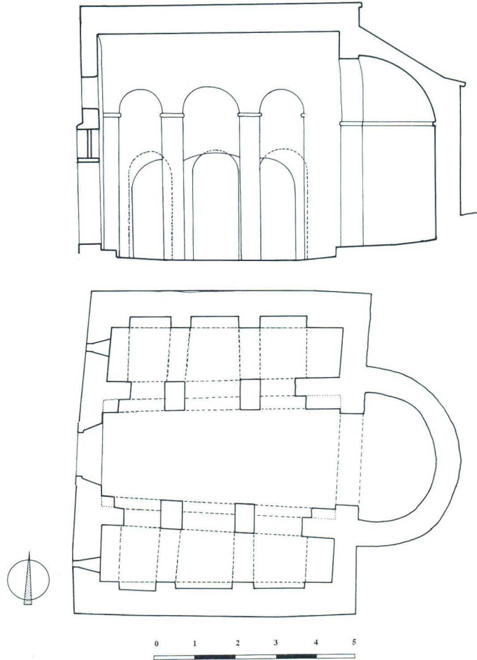
Izgled Sv. Duha nakon ranosrednjovjekovnog preuređenja
