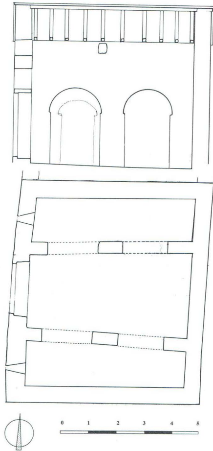
Pretpostavljeni izgled Sv. Duha iz 7. st. prema saznanjima najnovijih istraživanja
