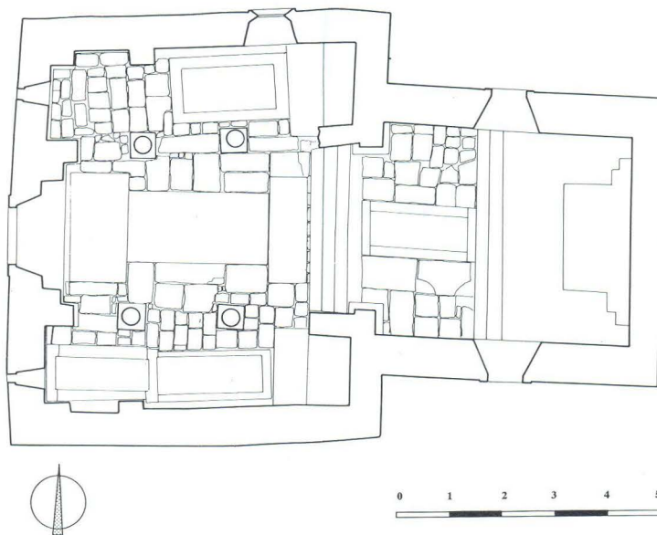
Tlocrt i uzdužni presjek Sv. Duha u Škripu, snimak postojećeg stanja
