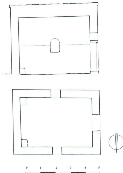
Pretpostavljeni izgled Sv. Ivana u Bolu iz 7. st. prema istraživanjima provedenim u toku radova 1984. g.
