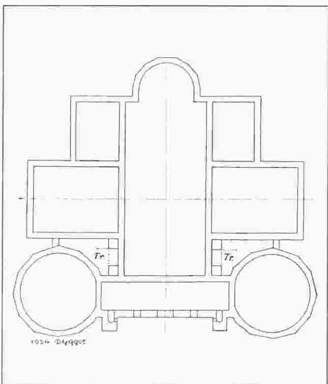
Slika 7. Tlocrt palače u rekonstrukciji E. DYGGVEA, 1954.
