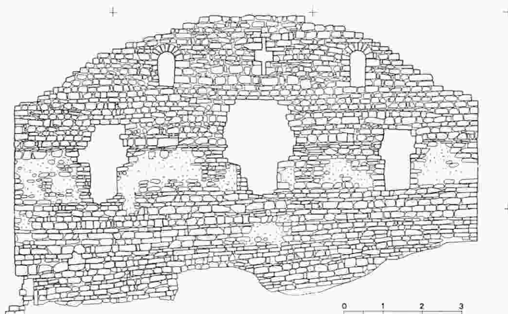
Slika 15. Fotogrametrija začelnog zida jugozapadne crkve (Dokumentacija Zavoda u Dubrovniku)
