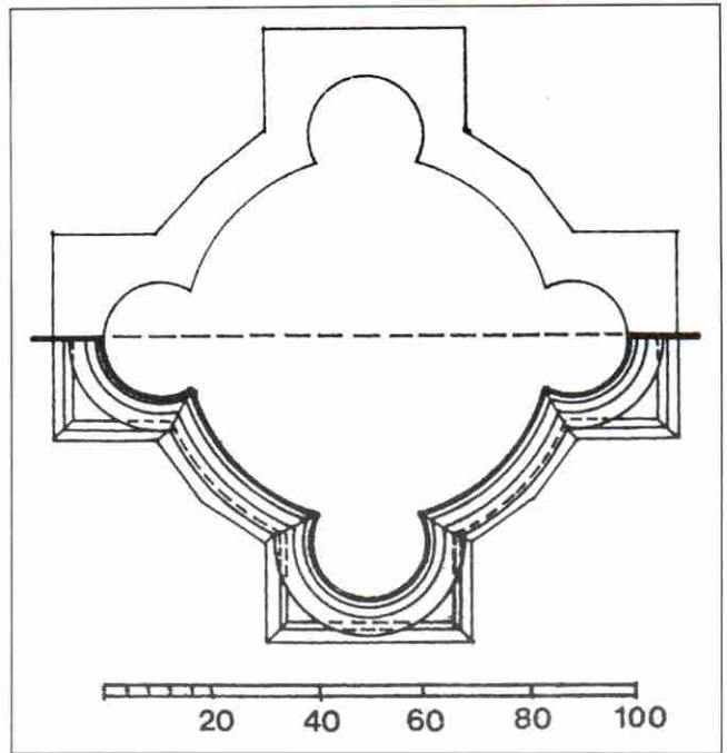
Slika 18. Topusko - presjek polustupa uz zapadno pročelje; uz njega je nacrtana zrcalno još jedna polovica, te je dobiven vjerojatni presjek stupova iz broda
