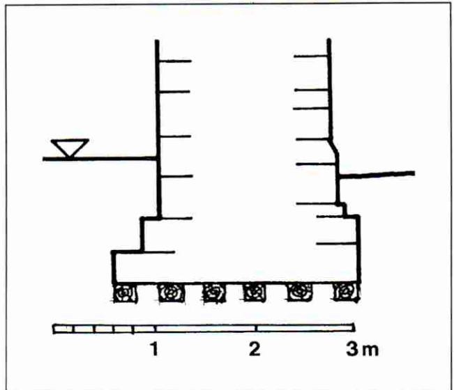
Slika 10. Presjek temeljne stope zapadnog pročelja cistercitske crkve u Topuskom - roštilj od drvenih greda ispod temelja nacrtan prema podacima S. SZAVITS-NOSSANA iz 1966.
