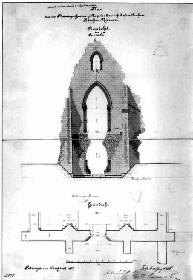
Slika 8. Topusko, cistercijski samostan - tlocrt i nacrt (zapadna strana) ostataka zapadnog pročelja (crtež F. ERBEN 1877., original u Planoteci Uprave za zaštitu kulturne i prirodne baštine Ministarstva kulture u Zagrebu)
