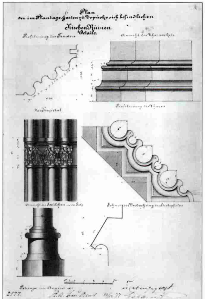
Slika 9. Topusko, cistercijski samostan - detalji zapadnog pročelja (prozor, portal, polustup u uglu, vijenac) (crtež F. ERBEN 1877., original u Planoteci Uprave za zaštitu kulturne baštine, Ministarstva kulture u Zagrebu).
