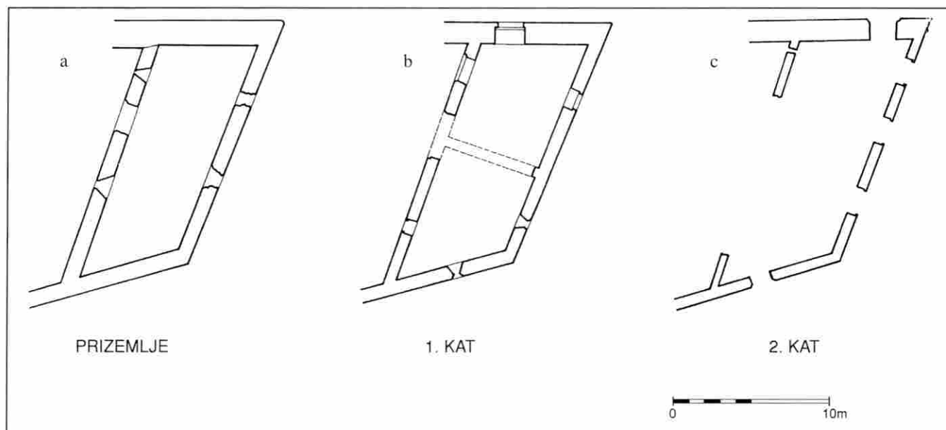
Slika 19. Tlocrt palasa: a) prizemlje, b) prvi kat, c) drugi kat
