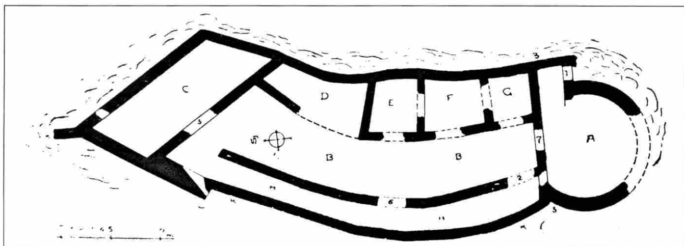
Slika 4. Tlocrt M. PILARA (1911.)
