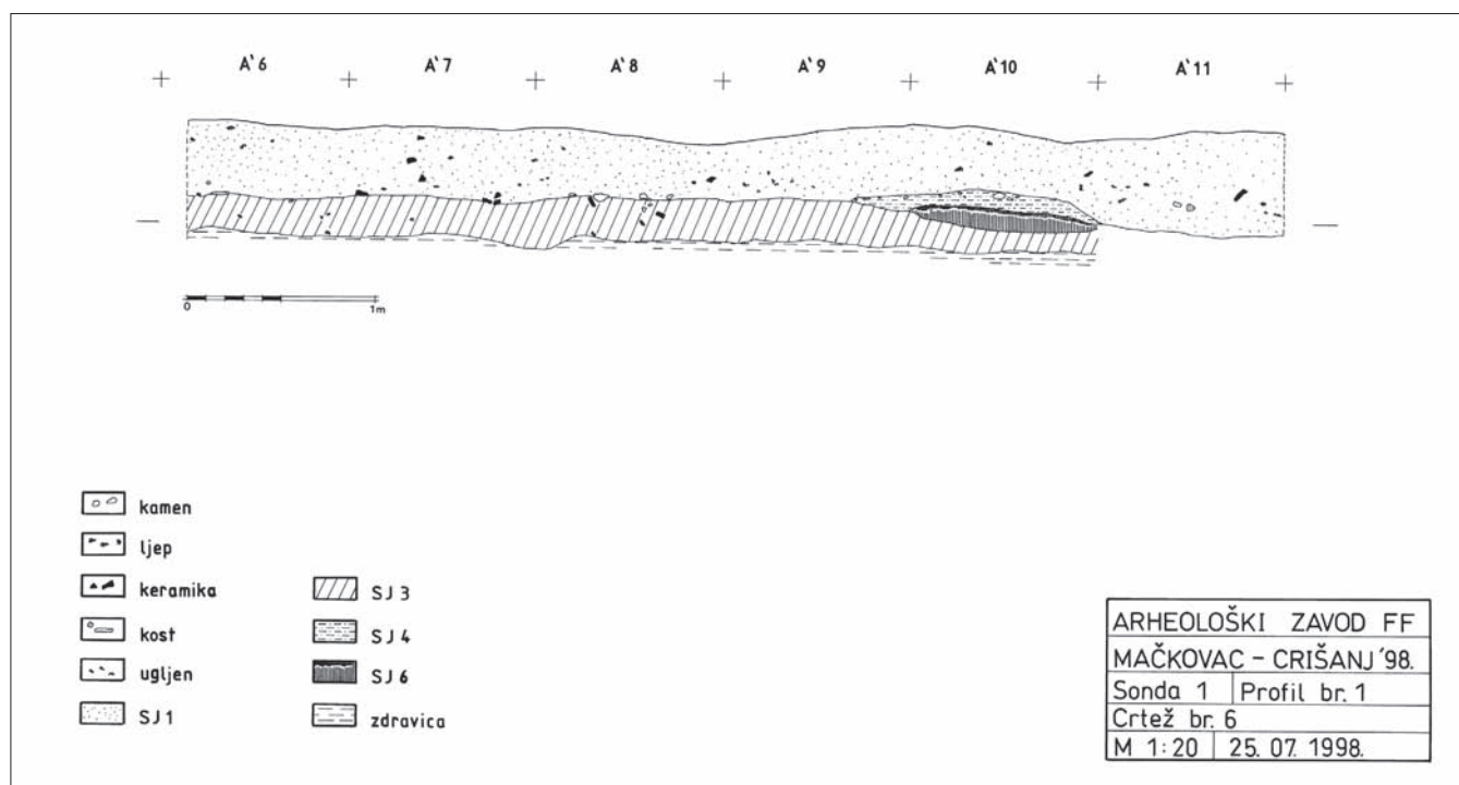
Sl. 3 Presjek ognjišta 1 (crtež: Marta Perkić)
