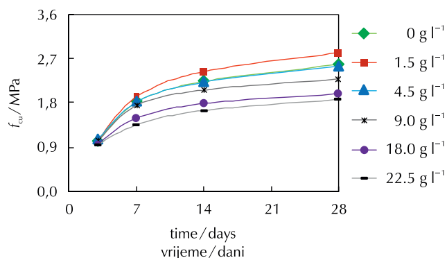
Fig. 3 – Relationship between the compressive strength of soils and time Slika 4 – Veza između tlačne čvrstoće tla i vremena
