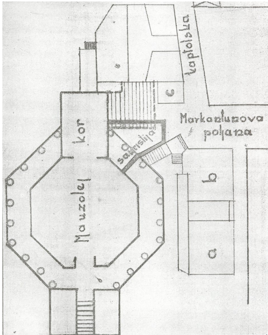
8. Plan pomicanja sakristije na jugoistočnoj strani katedrale. Debelom crtom označen je njen raniji položaj, a šrafirano polje jest mjesto gdje je 1938. godine ponovno sagrađena nakon rušenja stare. Time je otkriven dio periptera Dioklecijanovog mauzoleja sa stupovima.
