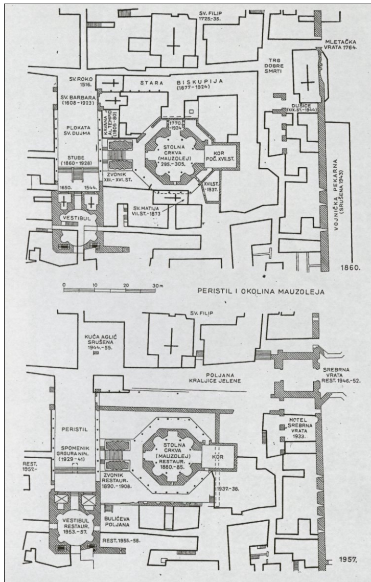
1. Tlocrt Dioklecijanovog mauzoleja u Splitu i njegove neposredne okolice. Na zgradama je označeno vrijeme njihove izgradnje i rušenja. Donji crtež predstavlja današnje stanje. (S. Muljačić).
