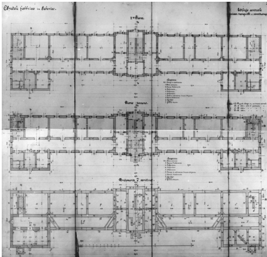
Bolnica u Šibeniku. Projekt K. Waidmanna središnjeg paviljona umobolnice za mirne bolesnike. Tlocrt prvog kata, prizemlja i podruma.
