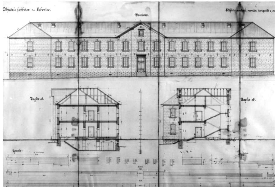
Bolnica u Šibeniku. Središnji paviljon umobolnice za mirne pacijente. Glavno pročelje i poprečni presjeci.
