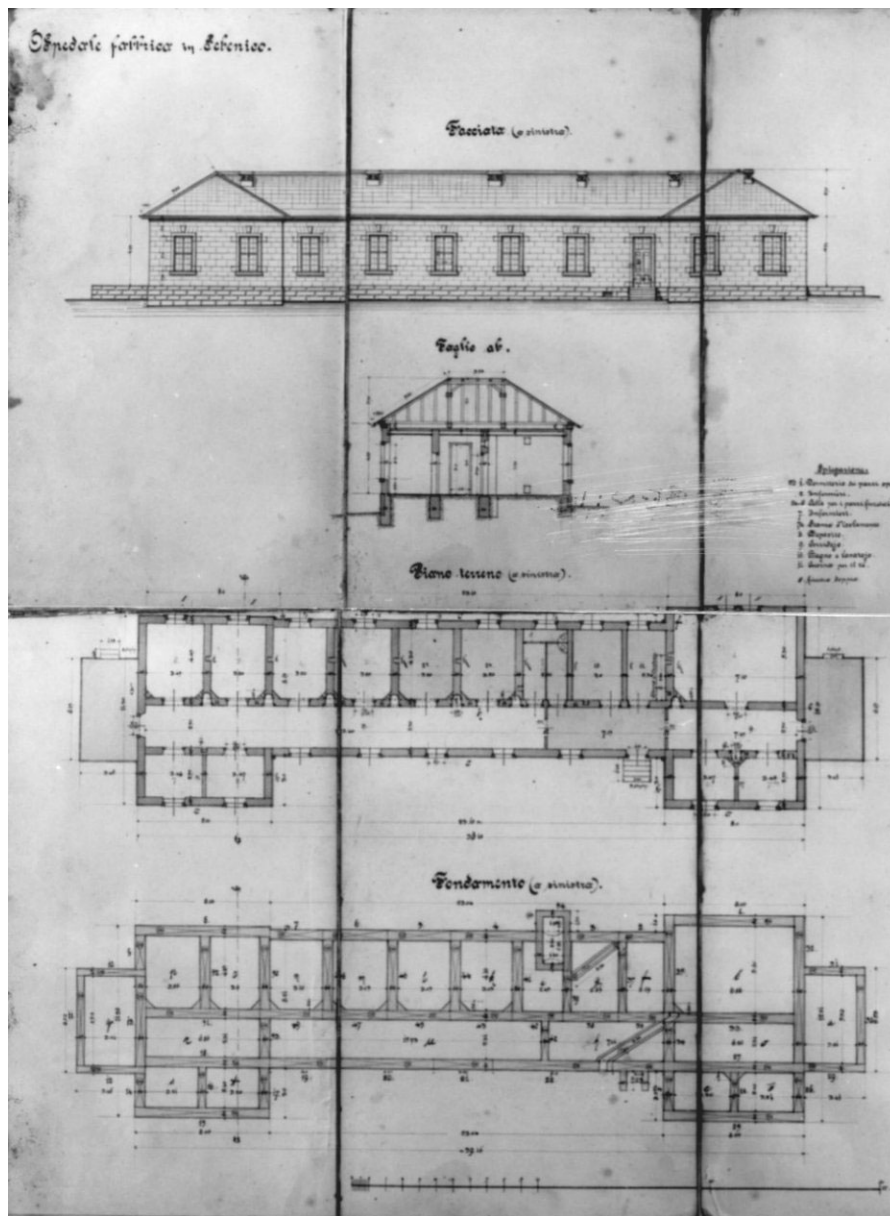
Bolnica u Šibeniku. Projekt paviljona umobolnice za prljave i bijesne pacijente. Glavno pročelje, poprečni presjek, tlocrti prizemlja i temelja.
