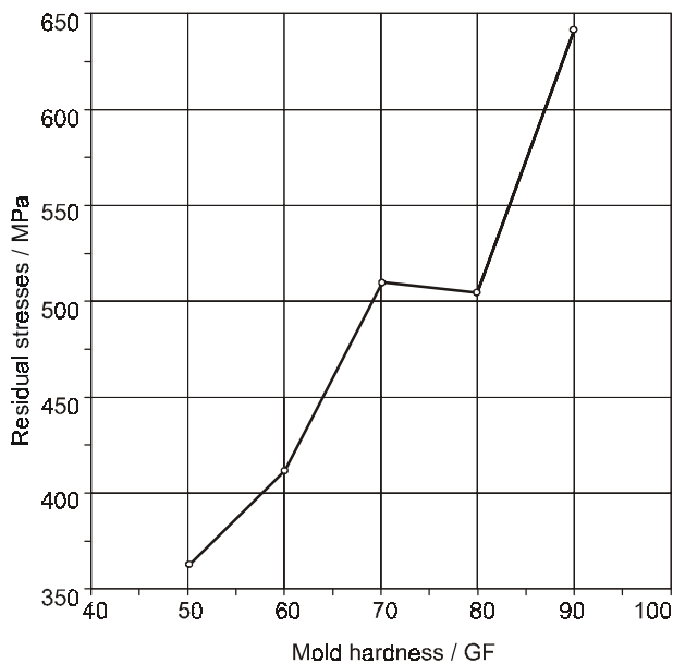
Figure 2. Dependence of residual stresses on mold hardness [4] Slika 2. Ovisnost zaostalnih naprezanja o tvrdoći kalupa [4]
