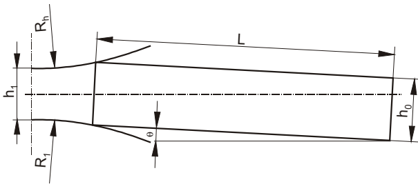
Figure 1. An exemplary design of a model of a charge and a tool Slika 1. Primjer projektiranja modela šarže i alata
