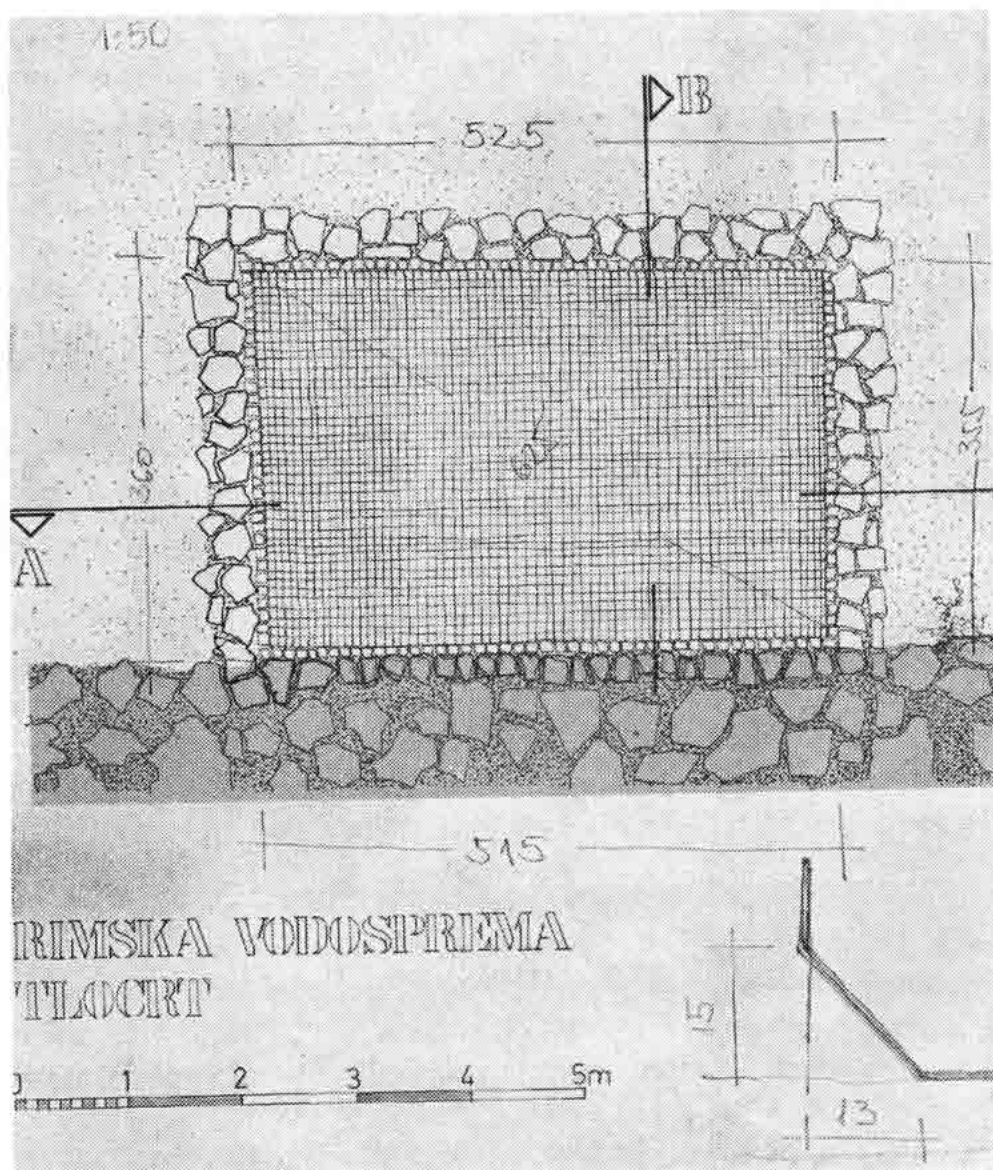
Sl. 58 — Tlocrt antičke vodospreme na »Steli«, snimila dipl. arh. Helena Knifić, 1976.
