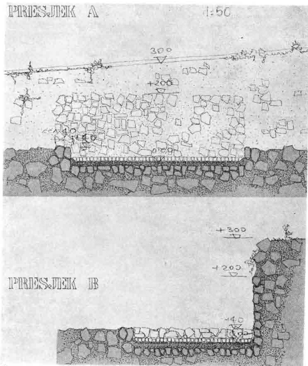
Sl. 59 — Presjeci A i B antičke vodospreme na »Steli«, dipl. arh. Helena Knjižić, 1976.
