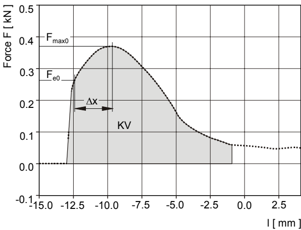
Figure 5. Bending loading diagram at v_2 = 5 \cdot 10^{-2} \text{ ms}^{-1} for steel DC 06 Slika 5. Dijagram savijanja pod opterećenjem pri brzini v_2 = 5 \cdot 10^{-2} \text{ ms}^{-1} za čelik DC 06
