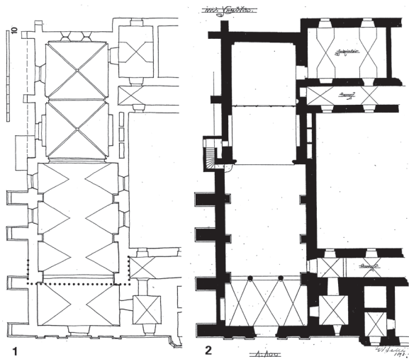
Sl. 5 Križevci – tlocrt bivše augustinske-franjevačke crkve, snimljene prije regotizacije 1892. godine: 1. tlocrt snimka crkve iznad parapeta prozora, s ucrtanim svodovima (prikazane su i službe kod gotičkog svoda u svetištu), točkama je označeno vjerojatno protezanje srednjovjekovnog broda; 2. tlocrt ispod parapeta prozora, sa snimljenim vratima, stubištem na propovjedaonicu te ikonostasom u sredini svetišta (crtao H. Bollé)
