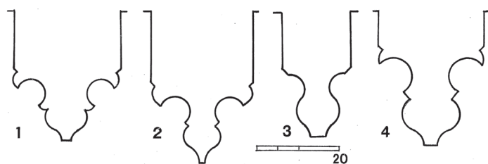
Sl. 18 Presjeci svodnih rebara nekih crkava u Slavoniji: 1. Zagreb, katedrala, svod južne apside; 2. Požega, crkva sv. Lovre, svetište; 3. Zagreb, katedrala, sakristija; 4. Zagreb, franjevačka crkva, svetište (skica) (crtao Z. Horvat)
