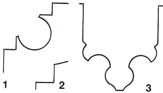
Sl. 14 Detalji svođenja svetišta bivše augustinske crkve, danas grkokatoličke katedrale Presvetog Trojstva: pojedinsti sustava svođenja, skice: 1. presjek polustupa u kutu svetišta; 2. profilacija zida uz svod; 3. presjek svodnog rebra u svetištu (crtao Z. Horvat)
