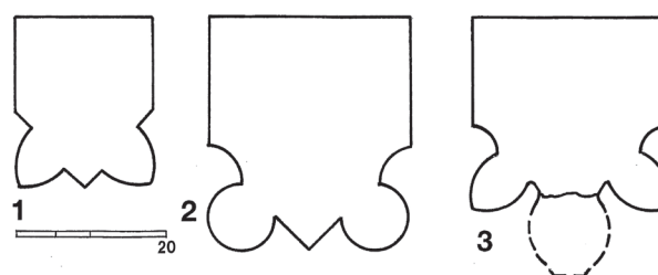
Sl. 17 Presjeci svodnih rebara nekih objekata 13. st. (crtao Z. Horvat): 1. Križevci, ulomak nađen uza sjevernu stranu grkokatoličke katedrale; 2. ulomak svodnog rebara, nađen na Medvedgradu; 3. ulomak svodnog rebara s našičke franjevačke crkve (prema R. Ivanušec, 2010.)
