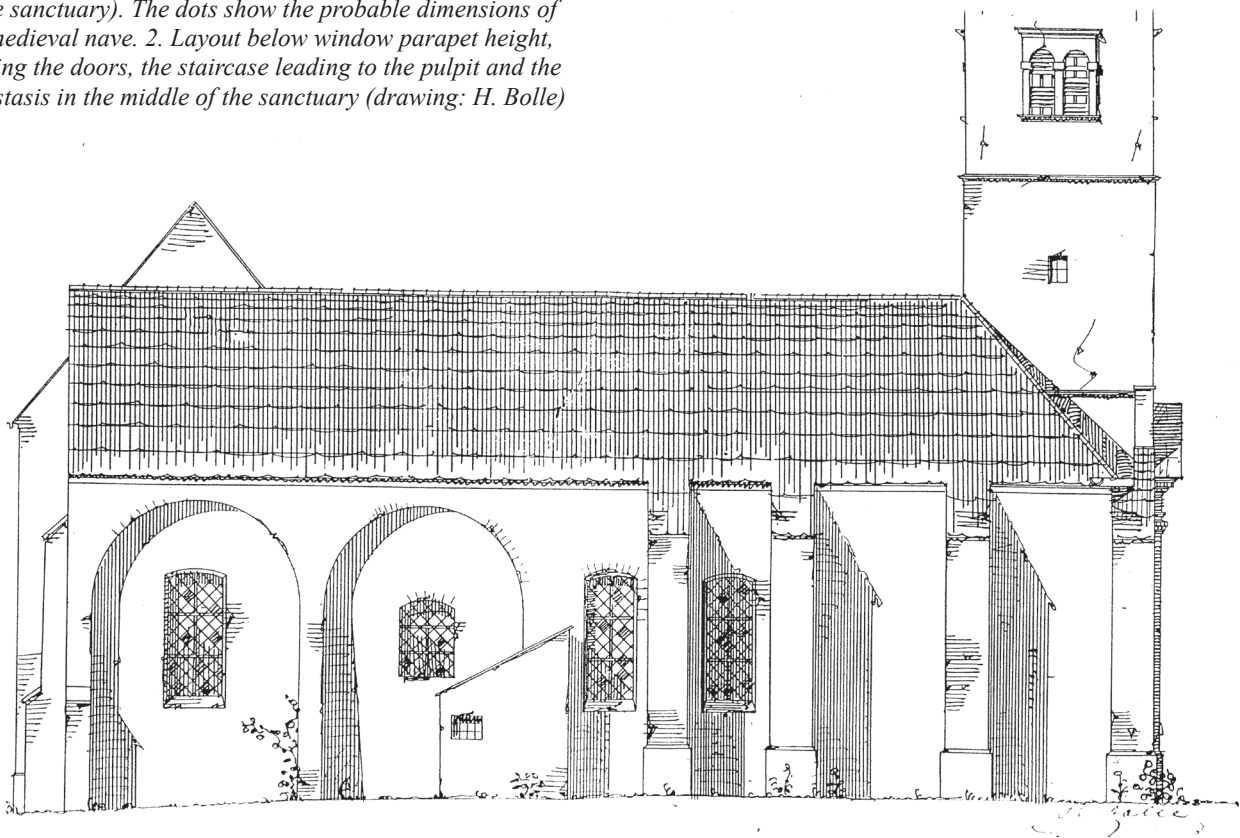
Sl. 6 Križevci – bivša augustinsko-franjevačka crkva – sjeverno pročelje (crtao H. Bolléa 1892. godine) Fig. 6 Križevci – former Augustinian/Franciscan church, northern facade (drawing: H. Bolle, 1892)
